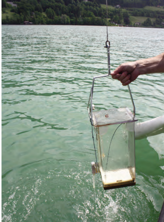
Abb. 6: Wasserschöpfer nach Schindler-Patalas, Foto: S. Wanzenböck.
