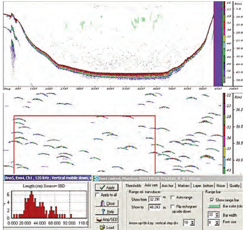
Abb. 14: Echogramm eines Transektes am Mondsee (14a, oben) und Ausschnittvergrößerung (14b, unten). Ganz rechts wird die Wassertiefe (R(m)) angezeigt. Das dunkelrote Band im oberen Übersichtsbild entspricht dem Seeboden, die kleinen Punkte stellen Fischechos dar. In der Ausschnittvergrößerung sieht man die Fischechos als bogenförmige Spuren. Die Echostärken (Dezibel, Negativwerte) sind farbcodiert und beziehen sich auf die Farbskala rechts. Ganz unten links wird die Größenstruktur der Fische dargestellt, welche aus den Echostärken berechnet wurde und sich auf die Fischechos im rot umrandeten Abschnitt der Vergrößerung beziehen.
