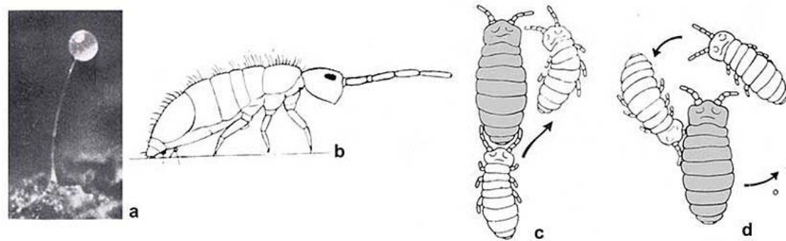
Abb. 2: Die von Schaller entdeckte indirekte Spermatophoren-Übertragung bei Collembola: a. Gestielte Spermatophore von Orchesella , b. Orchesella -Weibchen bei der Aufnahme einer Spermatophore, c. Podura aquatica : Ein Männchen (weiß) schubst das Weibchen von hinten und umläuft es anschließend, d. in der weiteren Folge setzt das Männchen mehrere Spermatophoren neben dem Weibchen ab und schiebt es dann in deren Richtung (verändert aus Schaller 1971).
