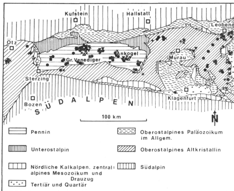
Abb. 3. Zeolithe in alpinen Klüften der Ostalpen. × Chabasit, ● Desmin, + Harmotom und Heulandit, ■ Skolezit, ▼ Thomsonit und Laumontit. Geologie vereinfacht nach BÖGEL & SCHMIDT (1976).
