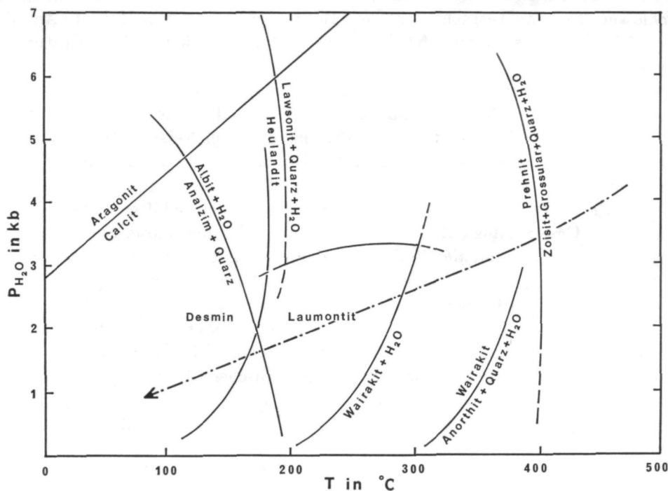
Abb. 4. p-T Diagramm nach LIU (1971c). Die strichpunktierte Linie gibt schematisiert den Trend der Mineralausscheidung in den alpinen Klüften der Ostalpen an
