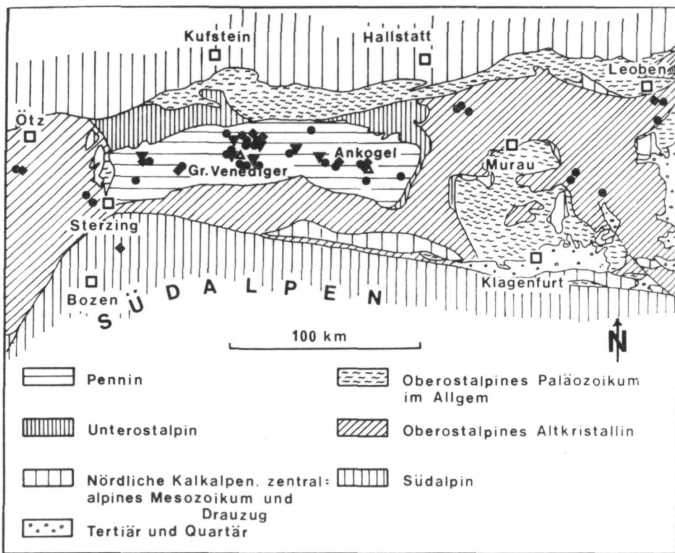
Abb. 2. Verteilung von Datolith, Prehnit und Apophyllit in alpinen Klüften der Ostalpen. ▼ Datolith, ● Prehnit, ◆ Apophyllit. Geologie vereinfacht nach BÖGEL & SCHMIDT (1976)
