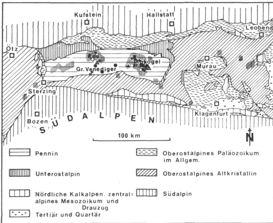
Abb. 1. Beryllium-Mineralien in alpinen Klüften und aus Pegmatitgängen der Ostalpen. \diamond Bavenit, + Bertrandit, \times Euklas, \blacksquare Gadolinit, \bullet Milarit, \blacktriangledown Phenakit. Die Vorkommen von Beryll sind durch eine enge Schraffur angedeutet. Geologie vereinfacht nach BÖGEL & SCHMIDT (1976)
