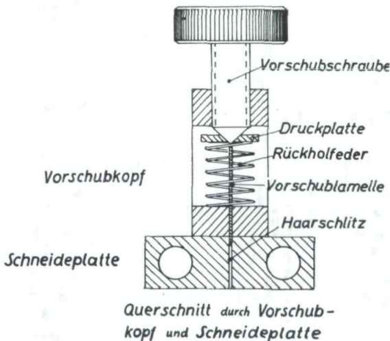
Abb. 2. Haarmikrotom nach BACHMANN & REUER.
