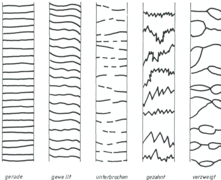
Abb. 5. Typen der Cuticulastruktur des menschlichen Kopffaars.
