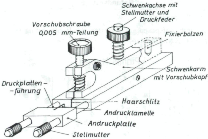
Abb. 1. Haarmikrotom nach BACHMANN & REUER.
