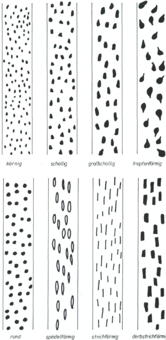
Abb. 3. Pigmenttypen des menschlichen Kopfhaares.
