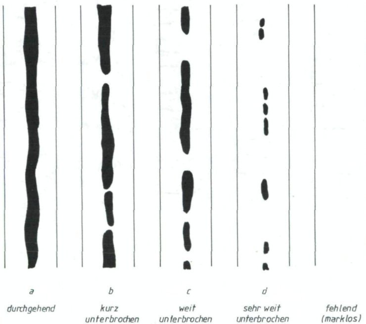
Abb. 4. Markstrangtypen des menschlichen Kopffaares.
