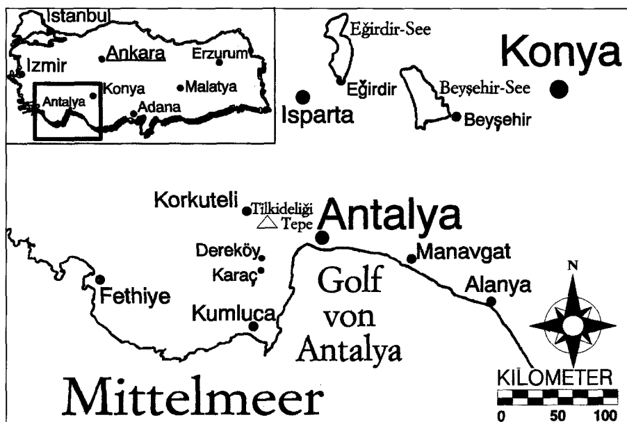
Abb. 1. Text-Fig. 1 Fundpunktkarte von ?Blastochaetetes astrocanalis nov. sp. und Genus et sp. indet. Form A in der Region westlich von Antalya. Sites of discovery of ?Blastochaetetes astrocanalis nov. sp. and Genus et sp. indet. Form A in the region west of Antalya.
