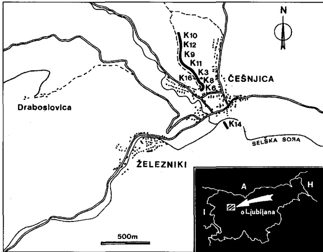
Abb. 1. Die Lage des Conodonten-Profiles Škovine (Ortschaft Železniki, West-Slowenien und der fündigen Probenpunkte K3, K6, K8, K10, K11, K12, K14 und K16.
