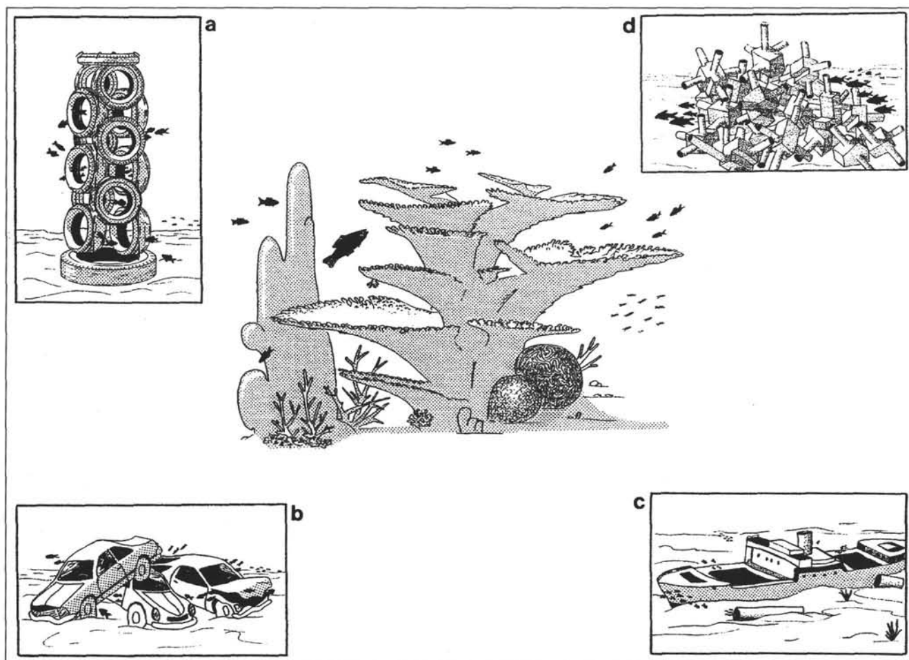
Abb. 6. Verschiedene Versuche, auf künstlichem Wege die Strukturvielfalt von Korallenriffen für Fischereizwecke nachzuahmen. a = „Reifenriff“ mit Stabilisierungsstangen; b = Autowracks; c = Schiffswrack; d = aufgetürmte Betonmodule.
