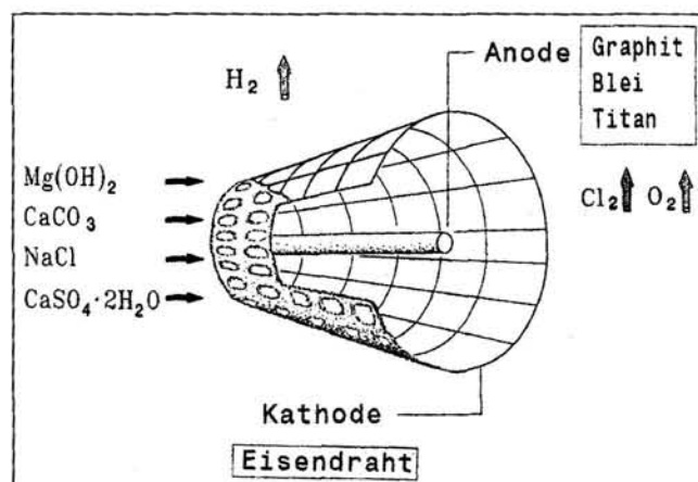
Abb. 3. Prinzip der elektrochemischen Abscheidung von Brucit, Kalk, Gips, Halit (Reihung nach Häufigkeit) auf dem als Kathode geschalteten Maschendrahtgerüst; an der Anode (aus Graphit oder Titan) entsteht gleichzeitig Sauerstoff und Chlorgas.
