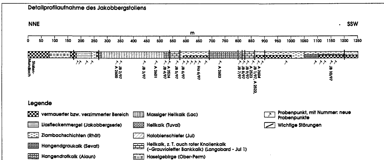
Abb. 4. Schematisches Stollenprofil des Jakobbergstollens, Lage der Proben und stratigraphische Einstufung der Schichtfolgen (aus GAWLICK & LEIN, 1997, geringfügig verändert und ergänzt). Zur Litho- und Mikrofazies sowie der stratigraphischen Einstufung der Proben siehe Tab. 1.
