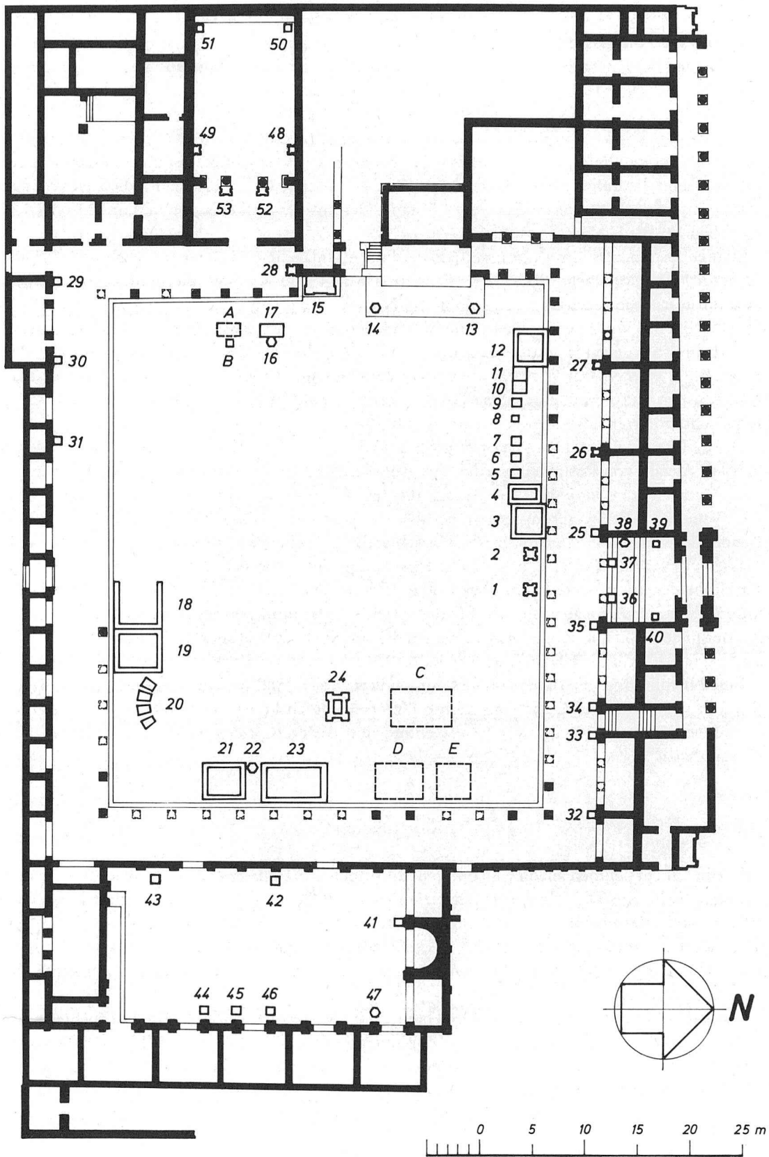
Abb. 16. Thamugadi, Plan des Forums (1:500).
