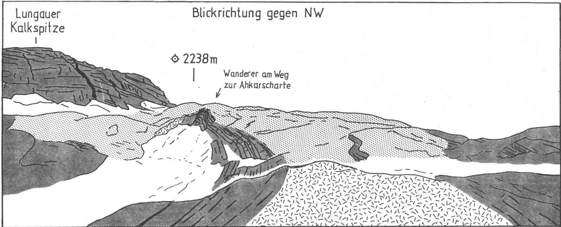
Abb. 16/2: Ansichtsskizze der Ostflanke der Lungauer Kalkspitze von einem Standpunkt etwa 200 m SE des Znachsattels. Dunkler, feiner Punktraster: Bänderkalke; Strichelsignatur: grobspätiger, bräunlicher Dolomit; lichter, grober Punktraster: massiger bis undeutlich gebankter heller Dolomit (Wettersteindolomit i.w.S.)
