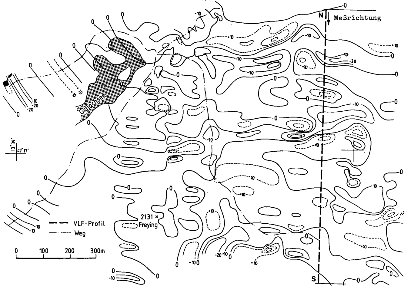
Abb. 16/6: Frasergefilterte Imaginärkomponente der VLF-Elektromagnetik im Gebiet Giglachsee-Vettertkar.
