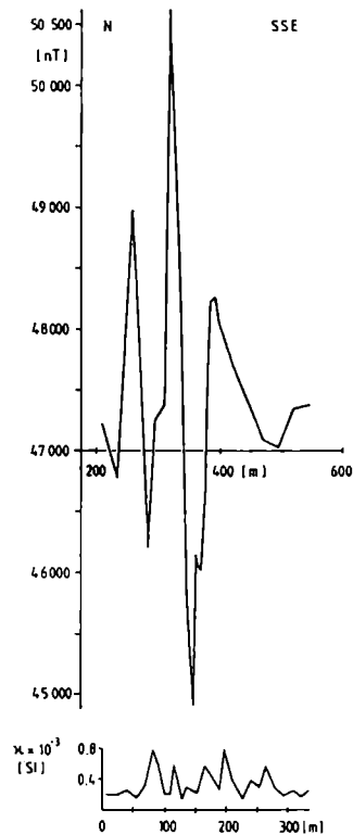
Abb. 16/8: Verteilung der Totalintensität (Blitzschlagmagnetisierung) im Vergleich mit insitut-Suszeptibilitätswerten am Rotmandlsitzkamm.
