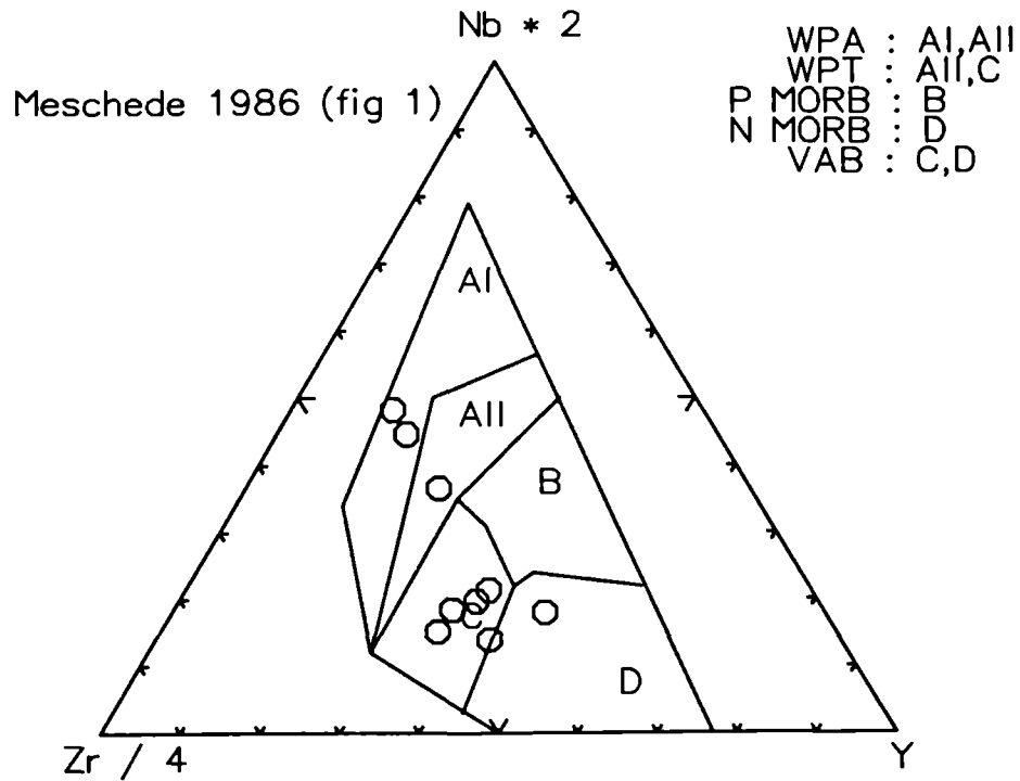
Abb. 5: Basaltdiskriminationsdiagramm nach M. MESCHEDA (1986) für die Amphibolite der Silvrettamasse (ÖK 144 Landeck).
