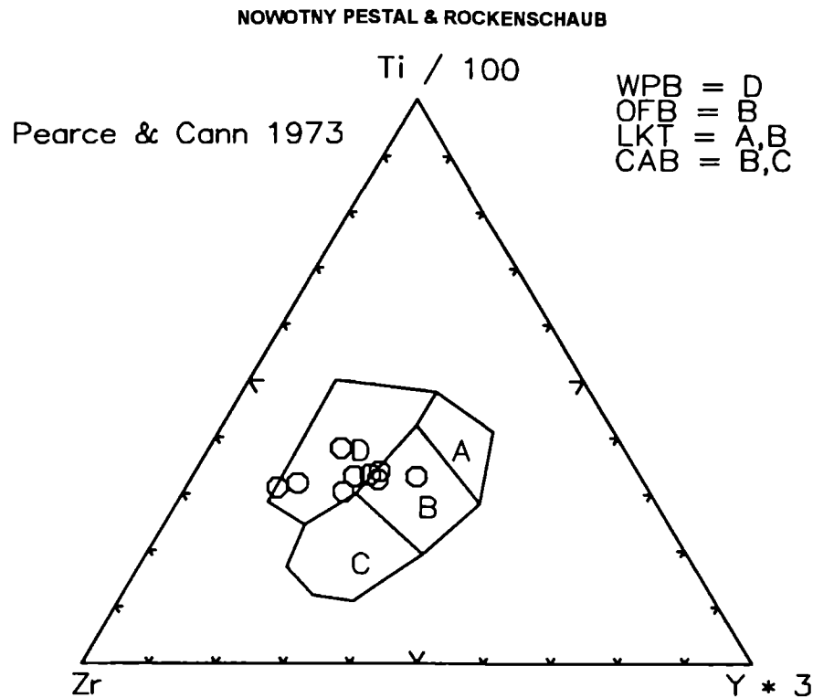
Abb. 6: Basaltdiskriminationsdiagramm nach J. A. PEARCE & J. R. CANN, 1973 für die Amphibolite der Silvrettamasse (ÖK 144 Landeck).
