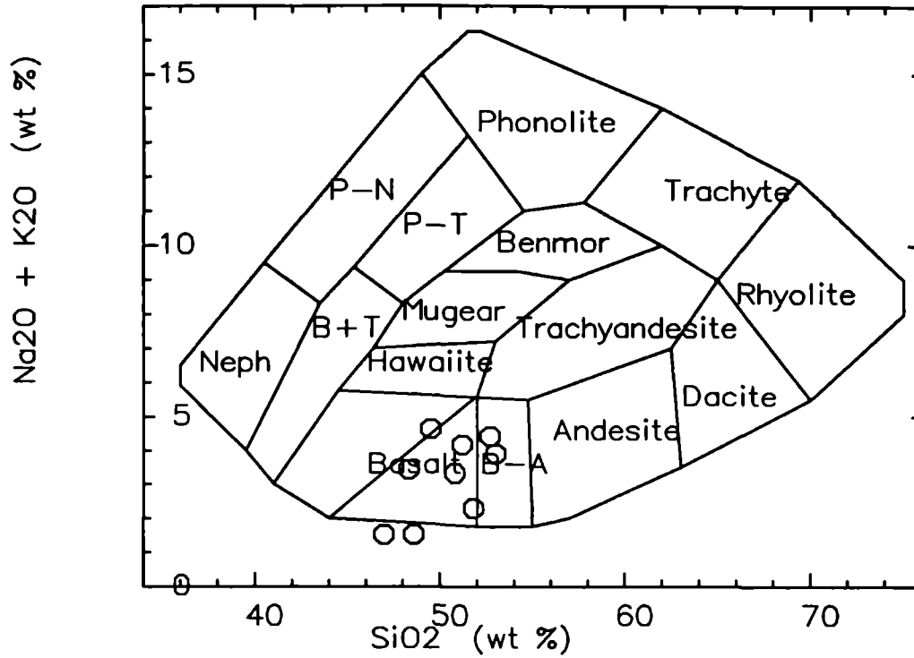
Abb. 4: SiO 2 - Na 2 O+K 2 O Variationsdiagramm nach K. G. COX, J. D. BELL und R. J. PANKHURST (1979) zur Einstufung von Vulkaniten mit Amphiboliten der Silvrettamasse (ÖK 144 Landeck).
