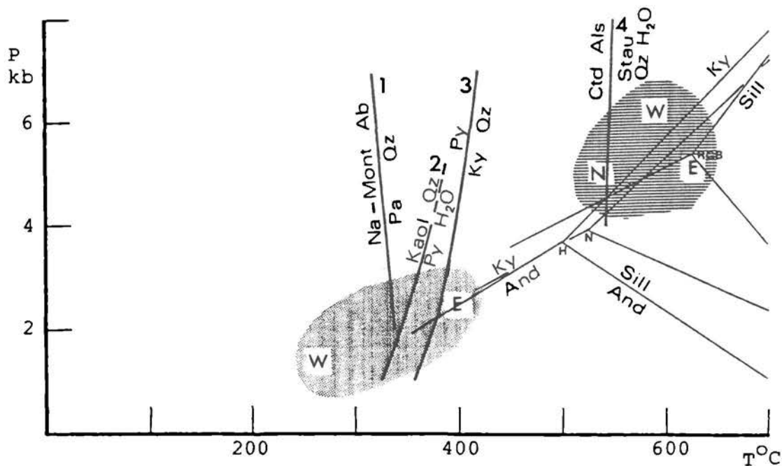
Abb. 4: Präalpine Metamorphose (Strichtraster) und Alpine Met. (Punktraster) im P-T-Diagramm; die Drücke sind nur grob geschätzt. Reaktionskurven: 1 CHATTERJEE (1973) 2 THOMPSON (1970) 3 HAAS & HOLDAWAY (1973) 4 HOSCHEK (1967, 1969); AlSi-Tripelpunkte nach NEWTON (1966), HOLDAWAY (1971) und RICHARDSON (1969)
