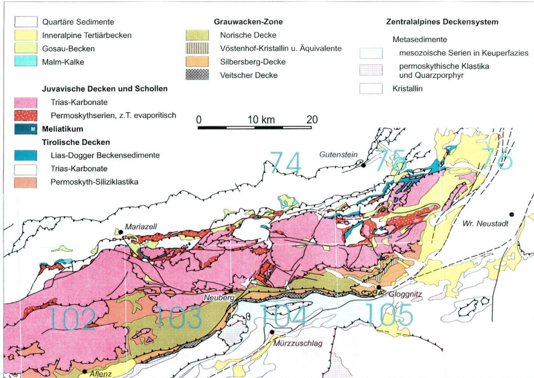
Abb. 1: Tektonische Übersicht der östlichen Kalkhochalpen
