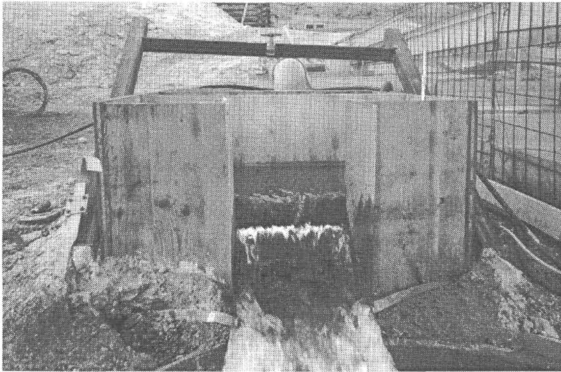
Abb. 7: Tunnel Semmering (Scheiteltunnel) - Meßkiste im Portalbereich Maria Schutz.
