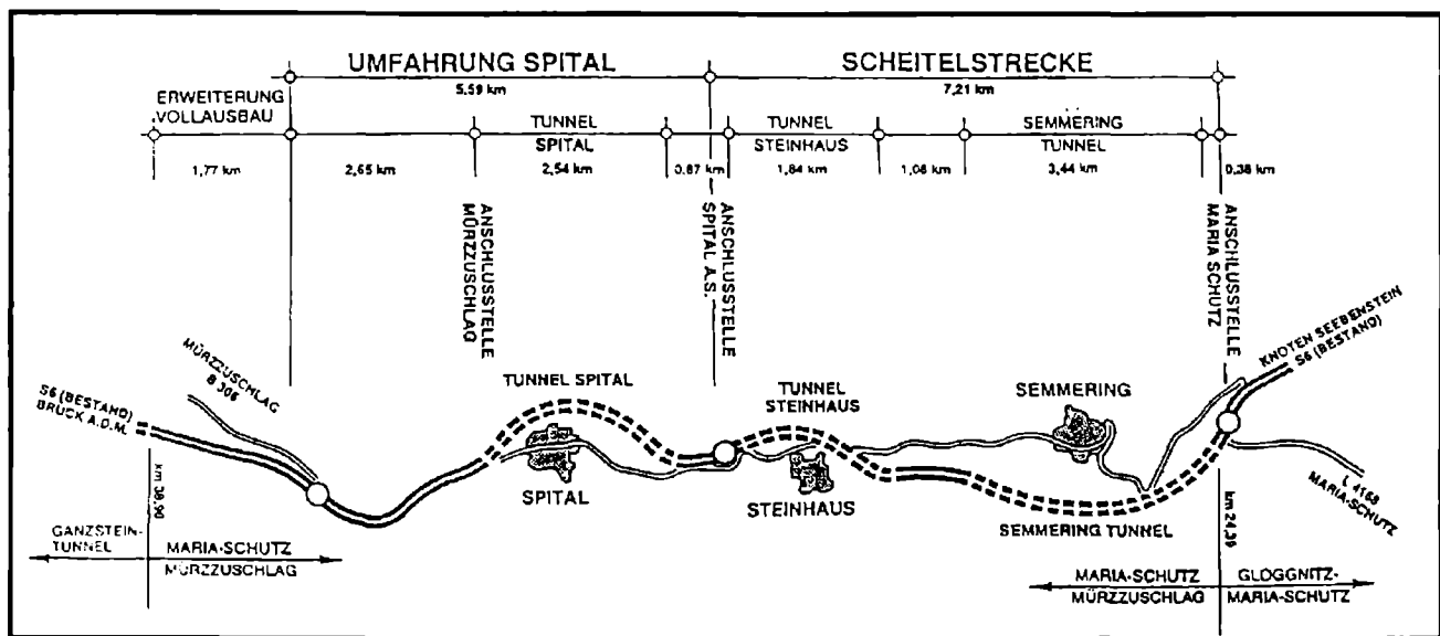
Abb.1: Übersichtslegeplan der drei Tunnelstrecken im Abschnitt des Lückenschlusses über den Semmering im Bereich Greis-Maria Schutz (NÖ.) und Grautschenhof (STMK).
