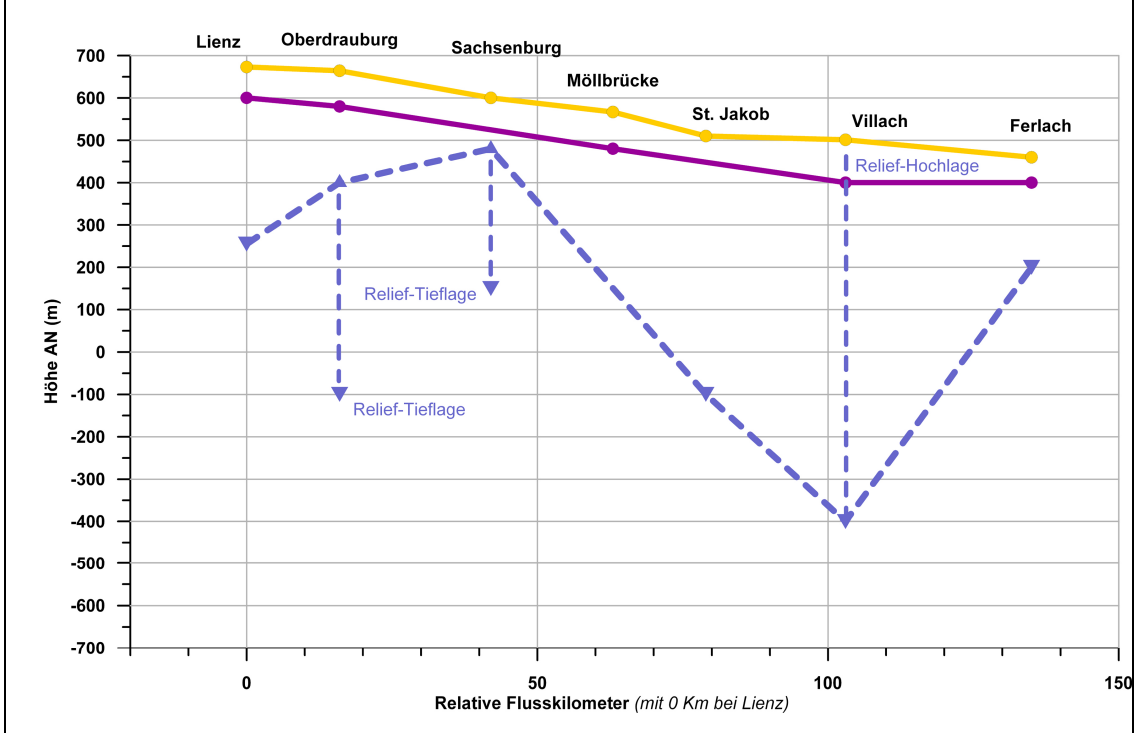
Abb. I: Geophysik im Drautal: Lage von lithologischen Grenzflächen
