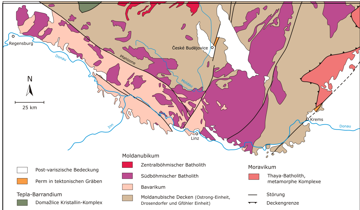
Abb. I: Tektonische Übersicht der südlichen Böhmischen Masse, verändert nach FIALA et al. (1995) und REITNER et al. (2006).
