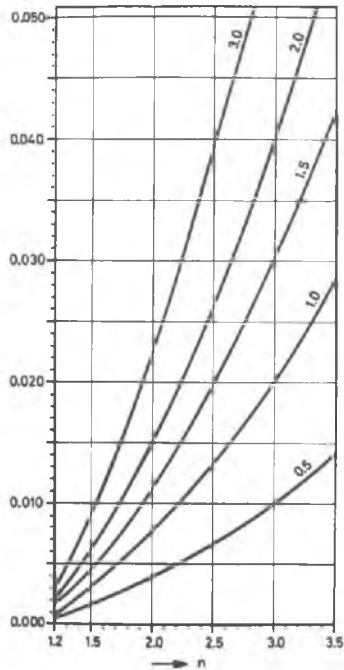
Abb. 2. Entstehende \pm Fehler (Ordinate) bei der Brechzahl n bei \pm Fehlern von 0,5; 1,0; 1,5; 2,0; 3,0 Relativprozent (Kurven) bei gegebenem n (Abszisse)
