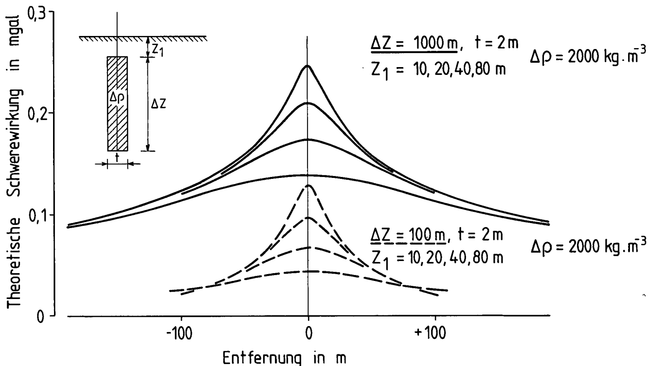
Abb. 1. Gravimetrische Störkörperberechnung, Plattenmodell.
