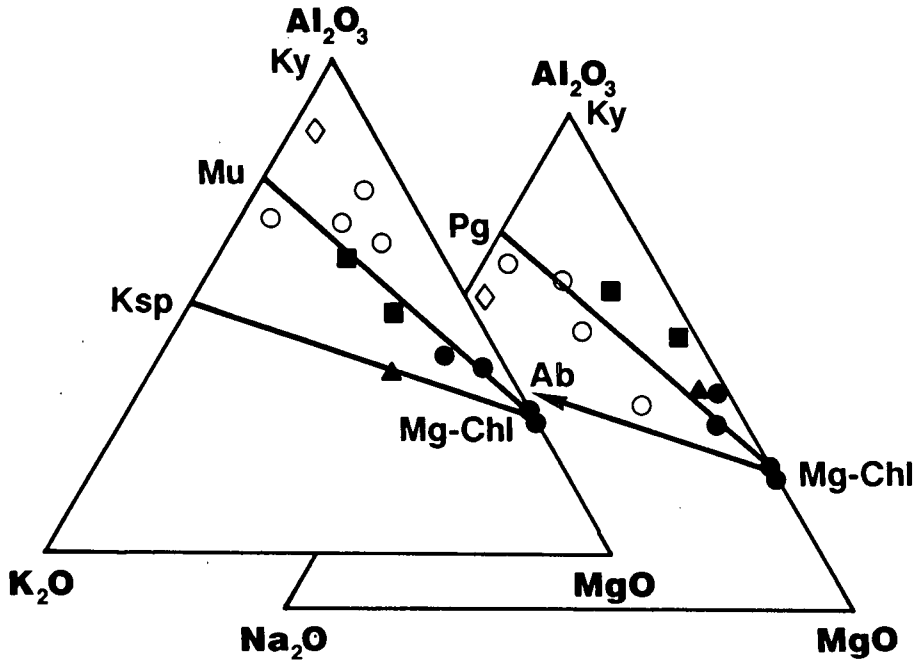
Abb. 3. Zusammensetzung der analysierten Proben im Al_2O_3 -MgO- K_2O bzw. Na_2O -Diagramm. Mit zunehmender Alteration nähert sich die Zusammensetzung dem Chlorit-Projektionspunkt. Legende siehe Tab. 1.
