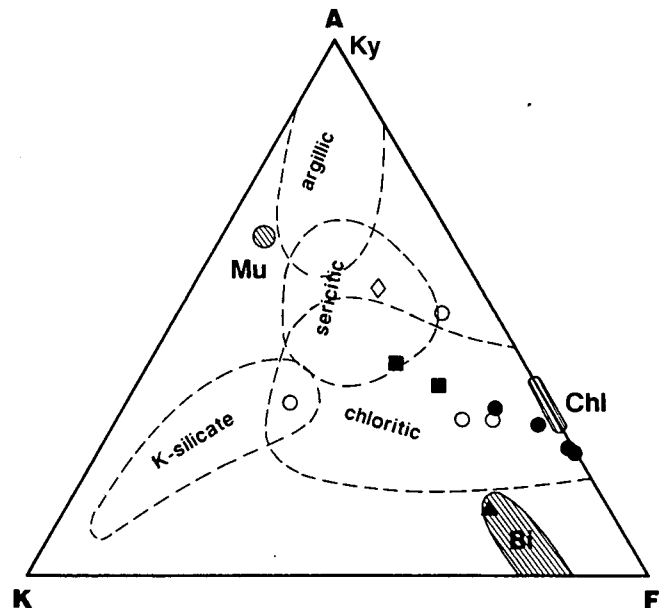
Abb. 4. A'KF-Diagramm für die analysierten Proben. Der Alterationsstil bei der Leukophyllitbildung entspricht einer Serizitisierung bzw. in einem fortgeschrittenen Stadium einer Chloritisierung. Legende siehe Tab. 1.
