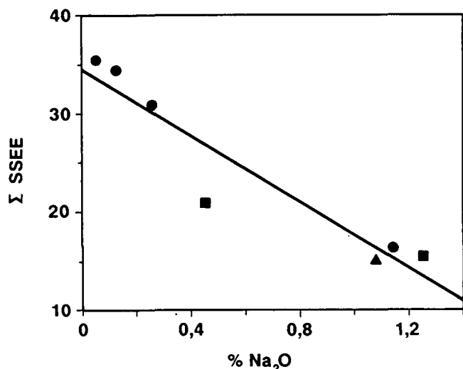
Abb. 5a,b,c. Mit zunehmender Alteration erfolgt eine relative Anreicherung der schwer mobilisierbaren Elemente (SSEE, Al) und des Mg. Leicht mobilisierbare Elemente wie z.B. Na werden aus dem System entfernt. Legende siehe Tab. 1.
