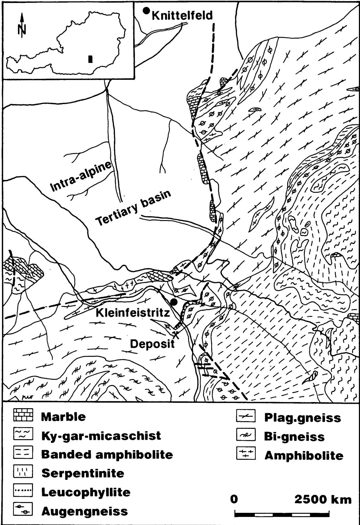
Abb. 1. Geologische Kartenskizze der Umgebung der Leucophyllitlagerstätte Weißkirchen.
