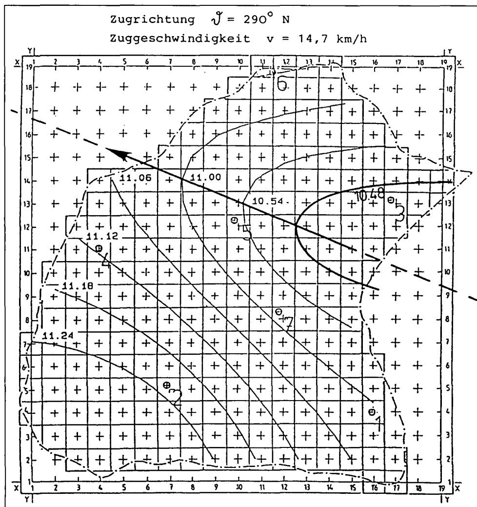
Abb. 7. Isochronenlinien für den Beginn eines Niederschlagsereignisses.
