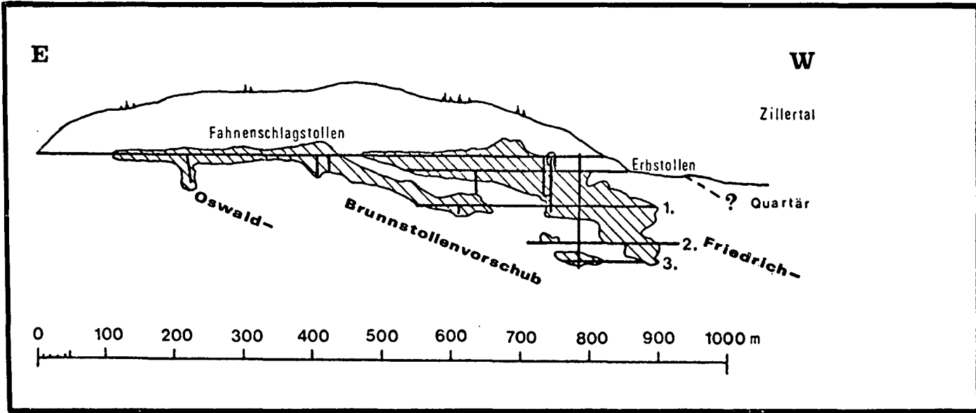
Abb. 1: Längsprofil des Friedrichlagers: der Hauptkunstschacht mit den drei Gezeugstrecken im Westfeld und den drei Adelsvorschüben nach dem Stand im Jahre 1867 (nach A. R. SCHMIDT, 1868; Taf. 1, Fig. 8).
