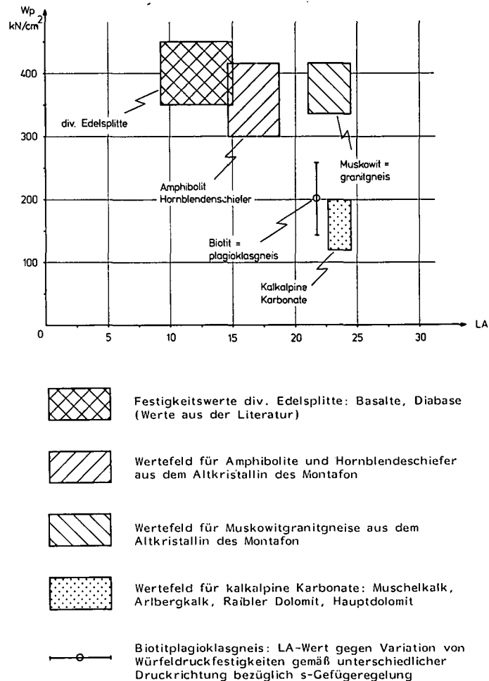
Abb. 2: Zusammenhänge zwischen Würfeldruckfestigkeit (Wp) und Los Angeles-Werten (LA).
