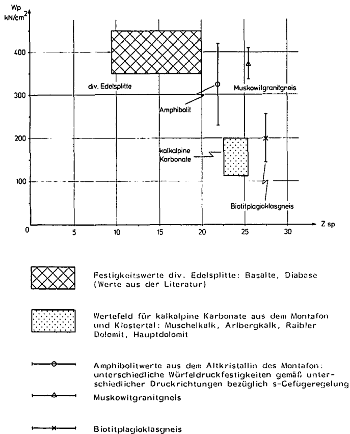
Abb. 3: Zusammenhänge zwischen Würfeldruckfestigkeit (Wp) und Schlagzertrümmungswerten (Z sp ).
