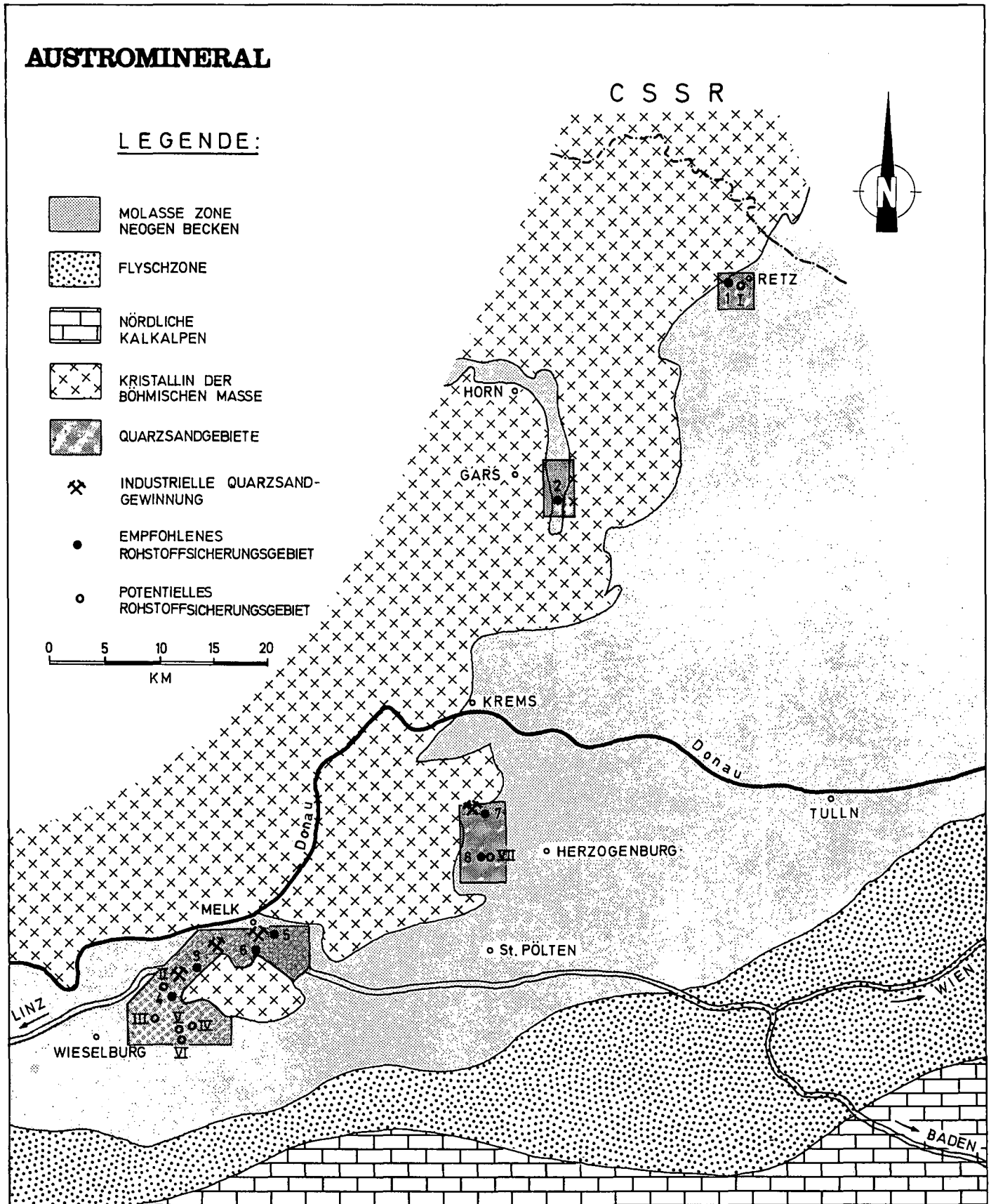
Abb. 1: Geologische Position der wichtigsten niederösterreichischen Quarzsandgebiete und Rohstoffsicherungsgebiete. Empfohlene Rohstoffsicherungsgebiete: 1 Diem, 2 Maiersch, 3 Hochstraßberg, 4 Gredinghof, 5 Wachberg, 6 Pöverding, 7 Kirchbühel, 8 Obritzberg-Winzing. Potentielle Rohstoffsicherungsgebiete: I Obernalb, II Rampersdorf, III Landfriedstätten, IV Geretzbach, V Rainberg, VI Grabenegg, VII Obritzberg-Ost.
