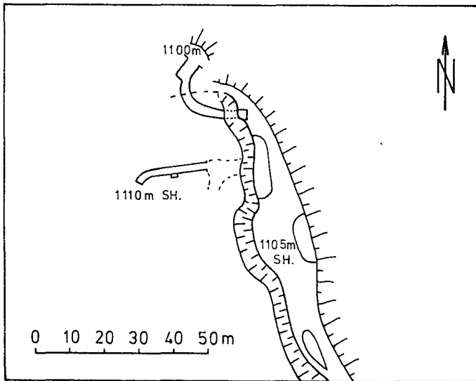
Abb. 2: Tagschürfe und Untersuchungsstollen am Lienz Schloßberg.
