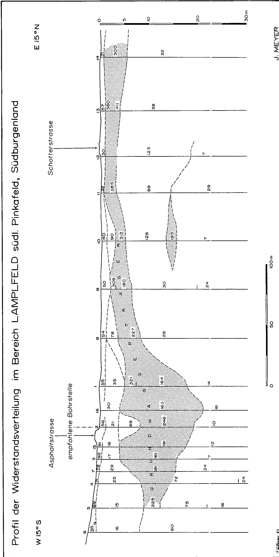
Abb. 10: Geoelektrische Tiefensondierungen entlang eines Talquerprofils westlich der Pinka (aus J. W. MEYER, 1984).
