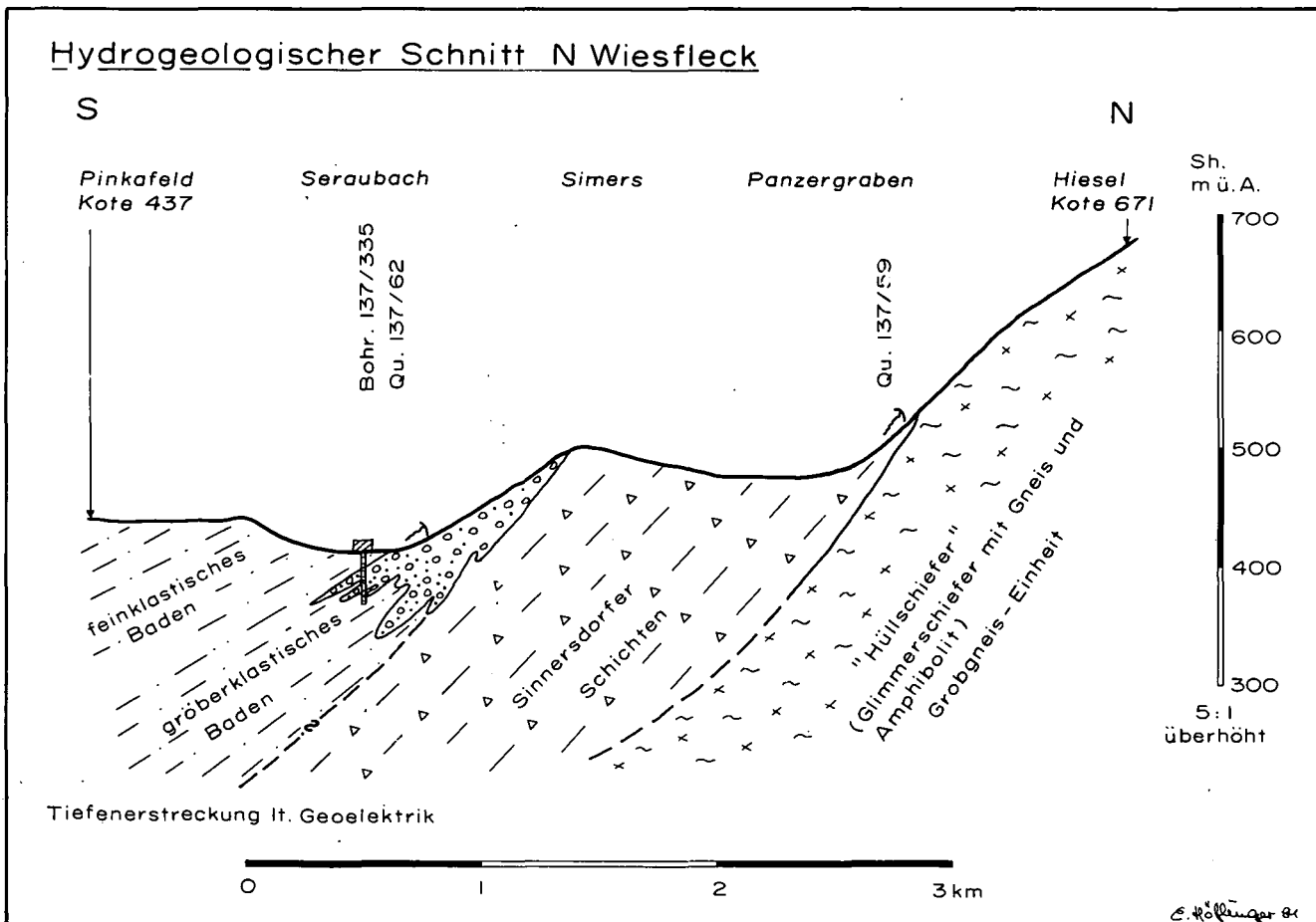
Abb. 8: Hydrogeologische Situation Pinkafeld – Wiesfleck mit Prognose für die Bohrung GBA-H: 137/335.
