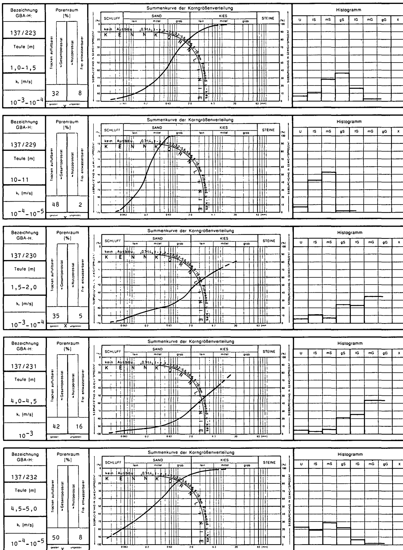
Abb. 7: Korngrößenverteilung, Durchlässigkeit und Porenraum (Erläuterungen im Text).
