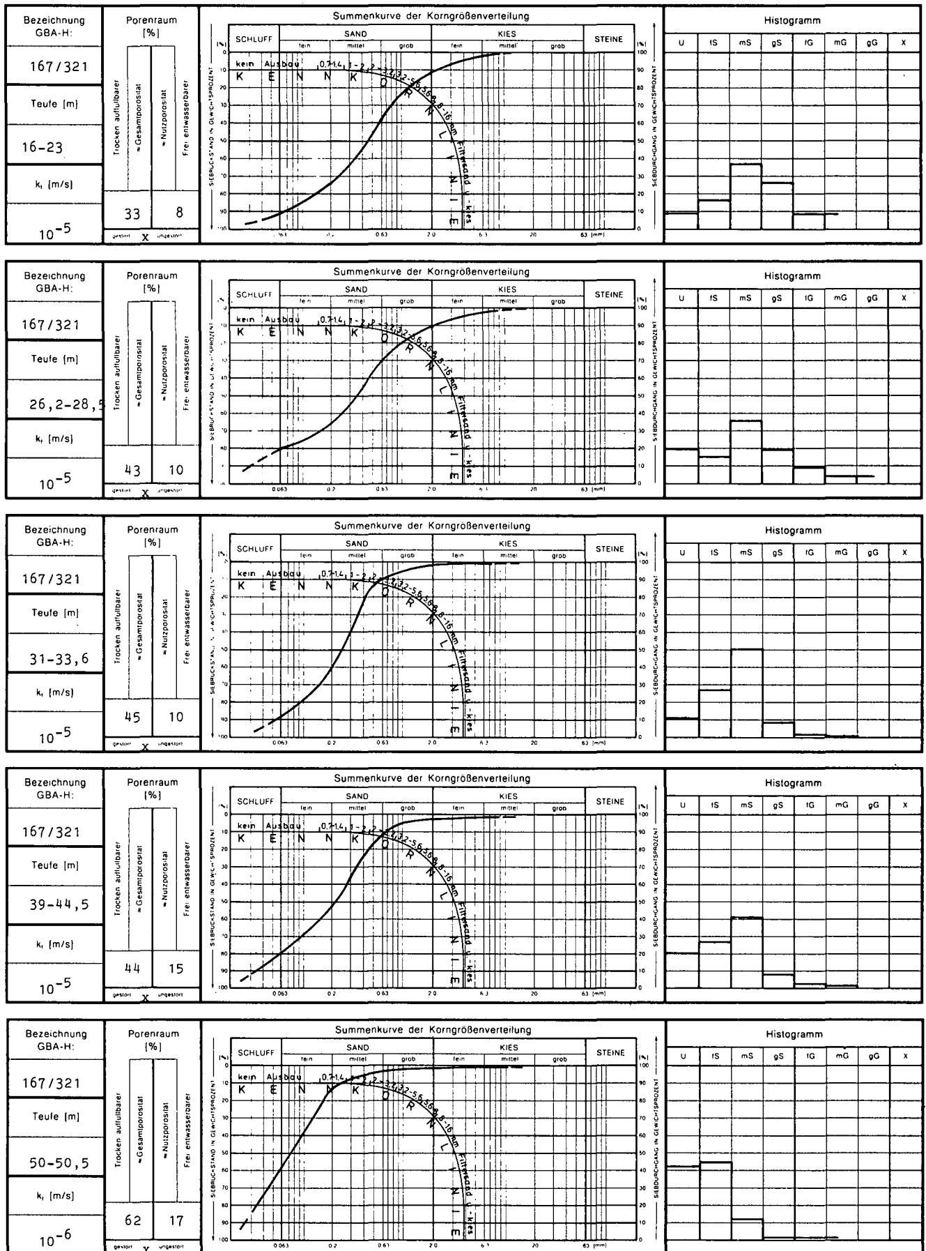
Abb. 4: Korngrößenverteilung, Durchlässigkeit und Porenraum (Bohrung „Neudauberg“, GBA-H: 167/321, MIL-Koordinaten: L 1034250, B 5226700).
