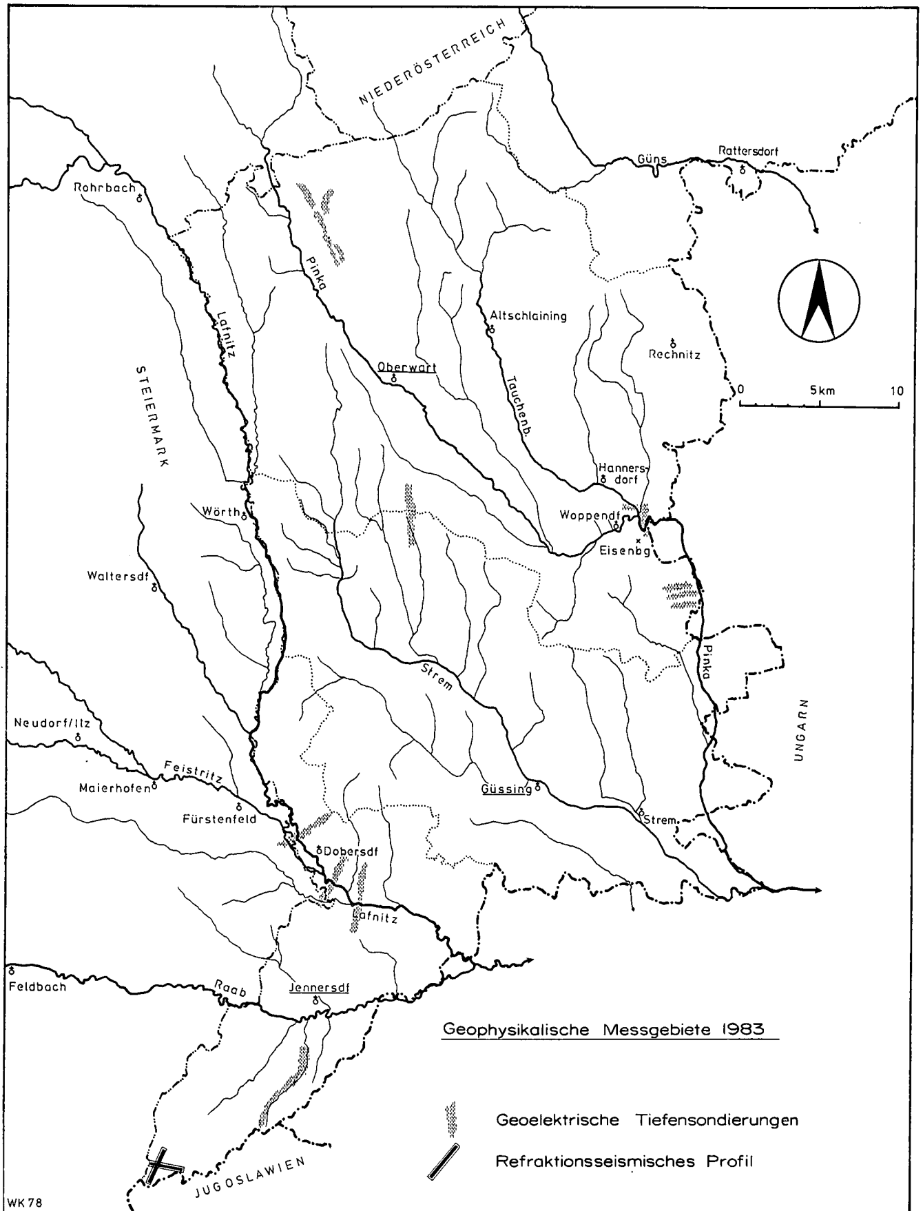
Abb. 1: Geophysikalische Meßgebiete.
