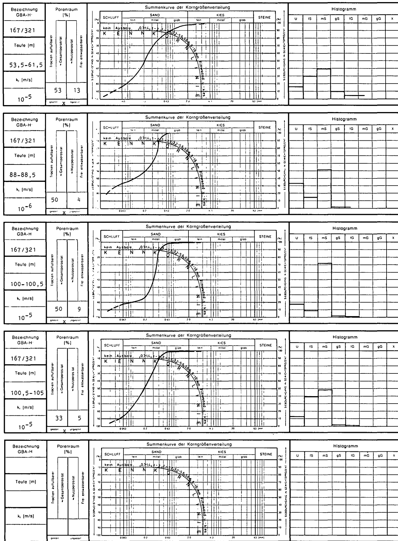
Abb. 5: Korngrößenverteilung, Durchlässigkeit und Porenraum (Bohrung „Neudauberg“, GBA-H: 167/321, MIL-Koordinaten: L 1034250, B 5226700).
