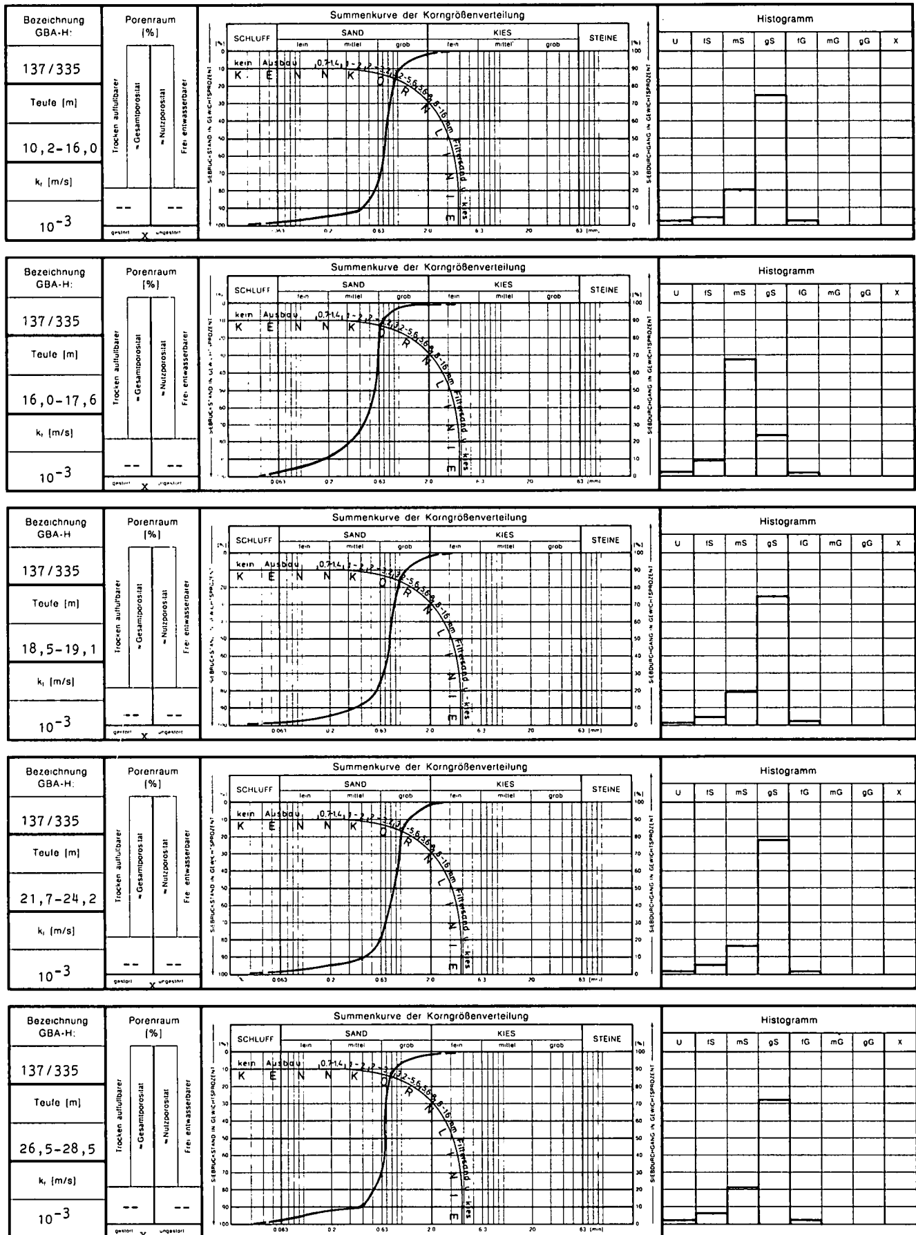
Abb. 9: Korngrößenverteilung, Durchlässigkeit und Porenraum (Bohrung „Wiesfleck“, GBA-H: 137/335, MIL-Koordinaten: L 1035000, B 5249850).
