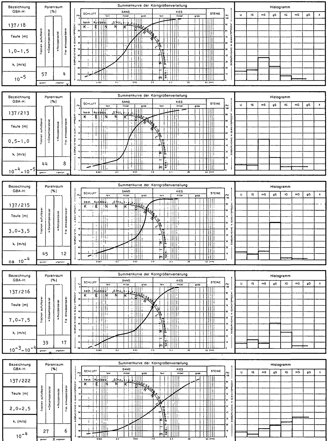
Abb. 6: Korngrößenverteilung, Durchlässigkeit und Porenraum (Erläuterungen im Text).
