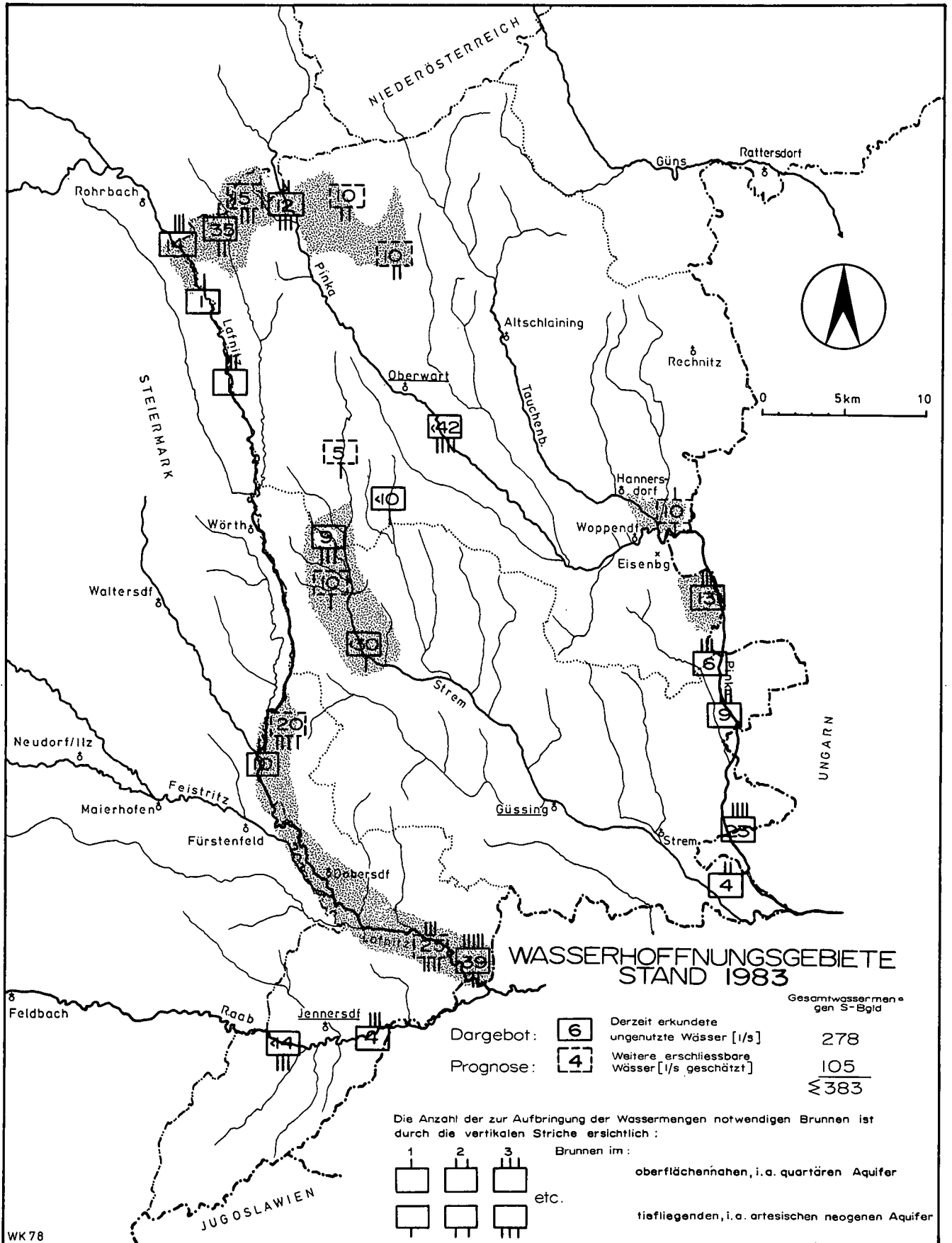
Abb. 11: Wasserhoffungsgebiete im südlichen Burgenland (Stand 1983).
