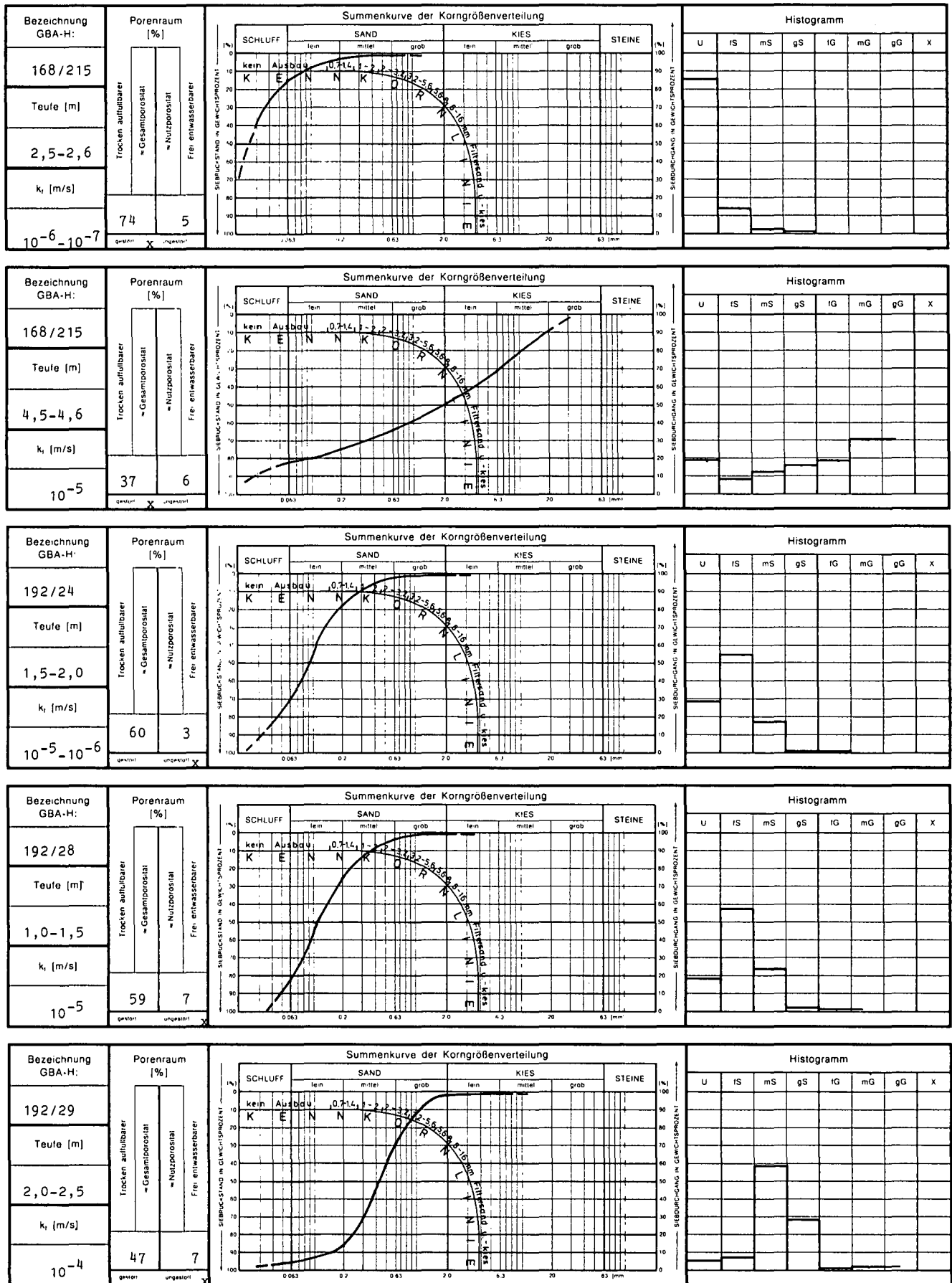
Abb. 3: Korngrößenverteilung, Durchlässigkeit und Porenraum (Erläuterungen im Text).
