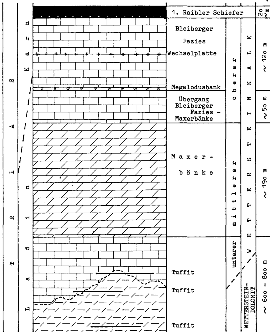
Abb. 1: Schichtfolge des Wettersteinkalkes von Bleiberg in maßstäblicher Darstellung vom 1. Raibler Schiefer bis zum 3. Tuffit im Liegenden.
