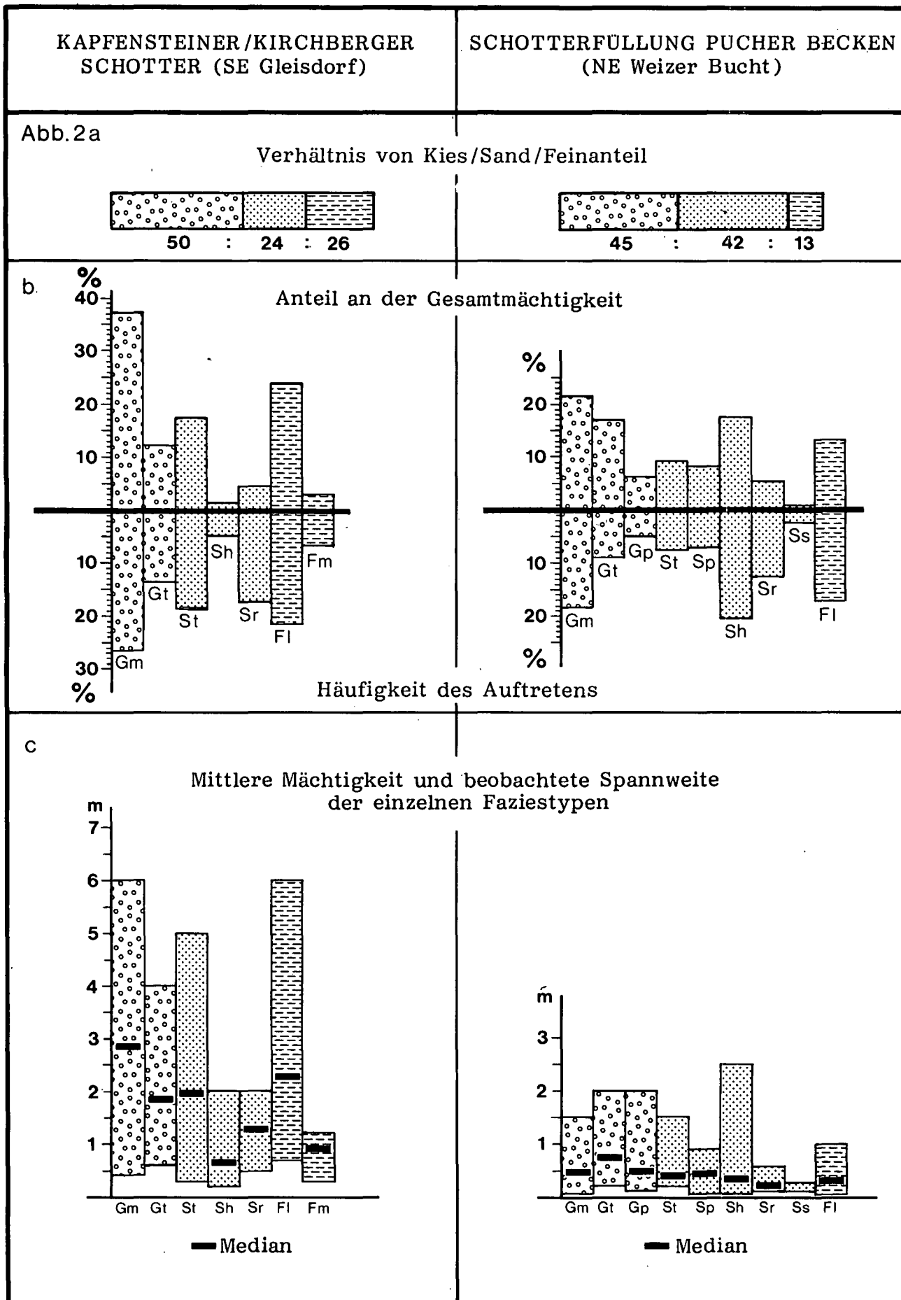
Abb. 2: Gegenüberstellung des sedimentologischen Aufbaus.
