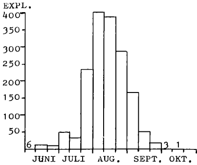
Noctua pronuba : Flugdiagramm 1980 für Deutschland
