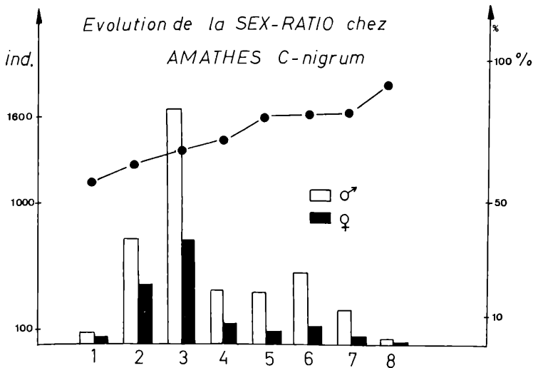
Figure 1: Evolution de la sex-ratio chez Amathes c-nigrum L.
