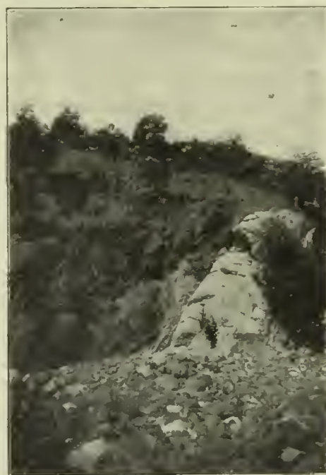
Fig. 3. Špala bei Këira; die Anticlinale des untertriadischen Kalkes, aus dem weicheren Schiefer hervortretend. (Nach Dr. F. Baron Nopcsa.)
