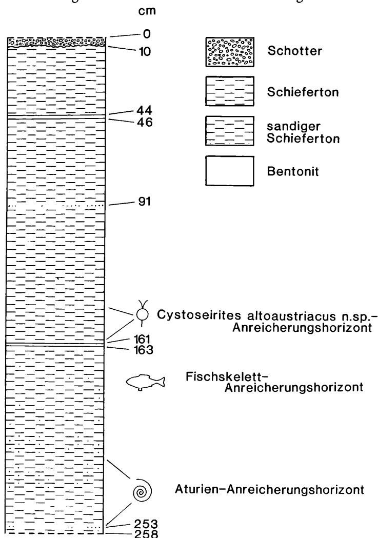
Abb. 4 Profil der hangenden Partien des Schiefertons im SW-Teil der Baugrube des Kraftwerkes Traun-Pucking.
