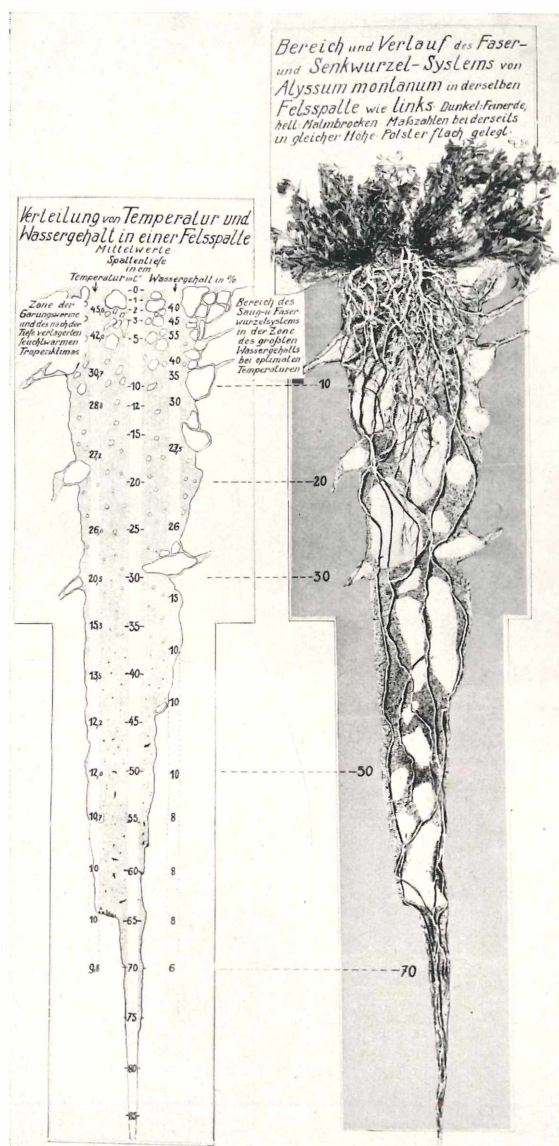
Fig. 9 Kombiniertes Längsschnittbild aus den Maßen von drei gleichartigen Spalten (Original in natürlicher Größe). Links: Mittelkolonne = absolute Tiefe der Spalte; linke Kolonne: Bodentemperaturen; rechte Kolonne: Wassergehalt in %. Rechts: Dieselbe Spalte mit der Anordnung des Faser- und Senkwurzelsystems von Alyssum montanum in natürlicher Anordnung darin. Orig. 1956.
