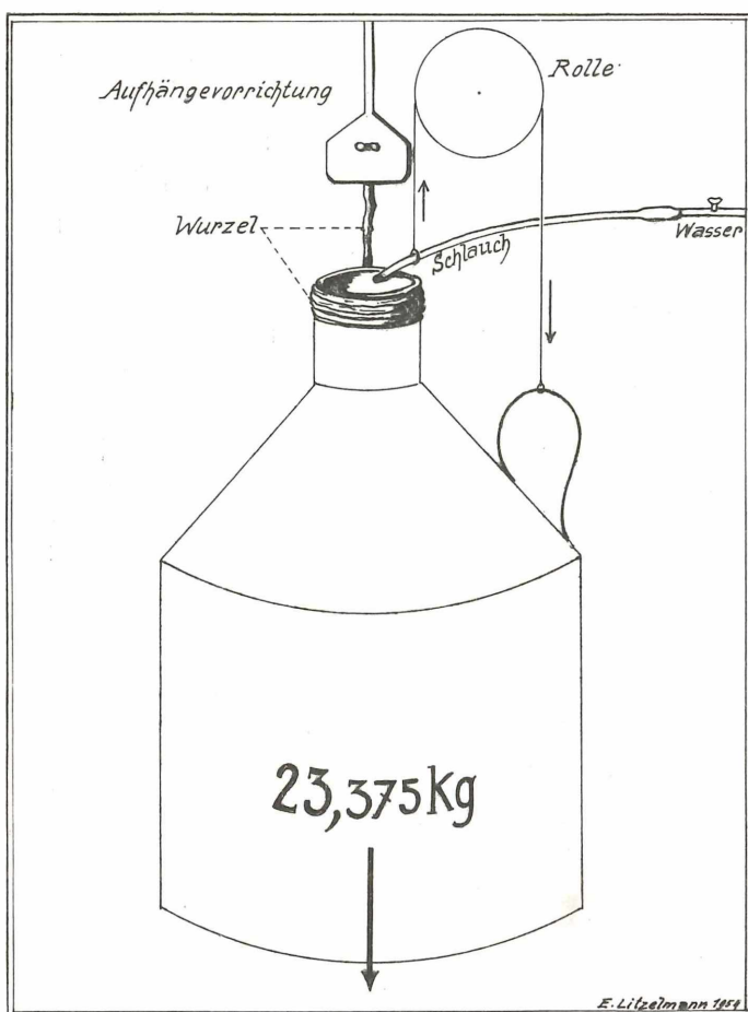
Abb. 9 Messung der Zerreifestigkeit einer Senkwurzel von Teucrium nontanum
