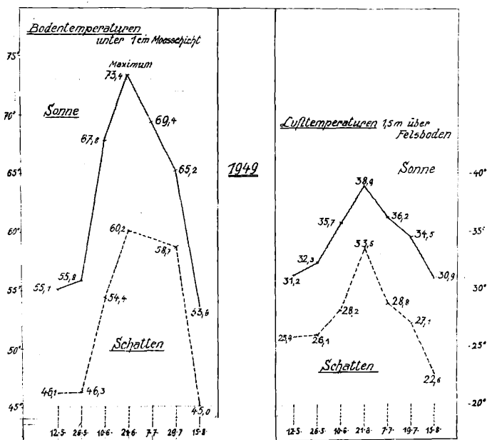
Abb. 3 Boden- und Lufttemperaturen auf dem Klotz im Dürresommer 1949 Orig. Litzelmann
