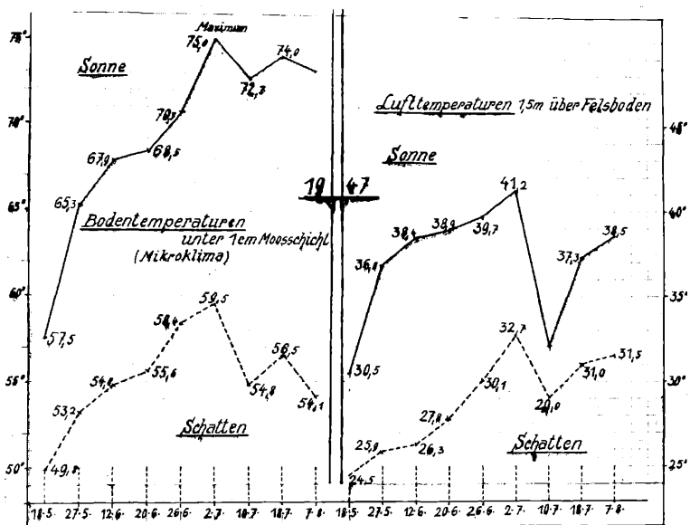
Abb. 2 Boden- und Lufttemperaturen auf dem Klotz im Dürresommer 1947. Orig. Litzelmann
