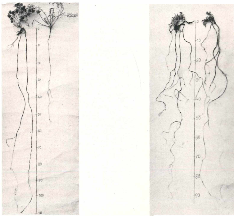
Fig. 8 Senkwurzeln einiger Spaltenbewohner vom Sporn des Isteiner Klotz. Von links nach rechts: Teucrium montanum , Euphorbia cyparissias , Potentilla arenaria , Globularia elongata . Litzelmann 1953.
