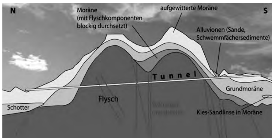
Abb. 3: Geologisch - tektonisches Profil längs des Umfahrungstunnels Henndorf, deutlich überhöht; Quelle: Sbg. Landesreg., Abt. 6/01 - Landesgeologischer Dienst
