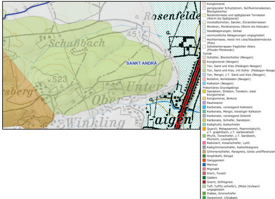
Abb. 11. Geologischer Kartenausschnitt Oberaigen. Dominierend sind Tone, Sande, Kiese und Kohle (Quelle Kagis Kärnten).
