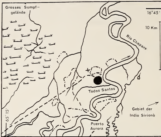
Abb. 1 Todos Santos am Rio Chapare und seine nächste Umgebung in Ostbolivien. Gestrichelte Linien: Urwaldstraßen und -pfade; Punkt-Strich-Linien: Pflanzungen; + Fundorte von Rivulichthys luelingi . (Zeichnung: Dr. K. H. Lüling)
