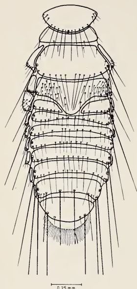
Abb. 11. Myrsidea splendidicola n. sp. ♀ dorsal
