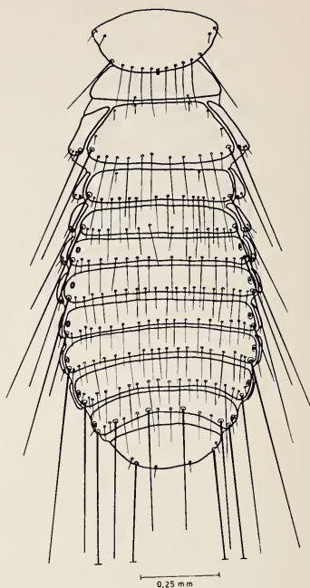
Abb. 12. Myrsidea splendidicola n. sp. ♂ dorsal
