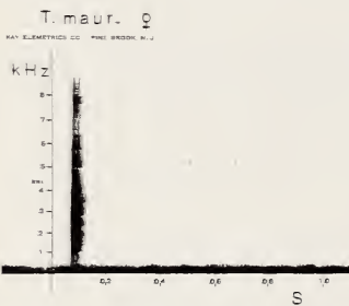
Abb. 8 (links): Einzelruf eines \varnothing von Tarentola mauritanica .
