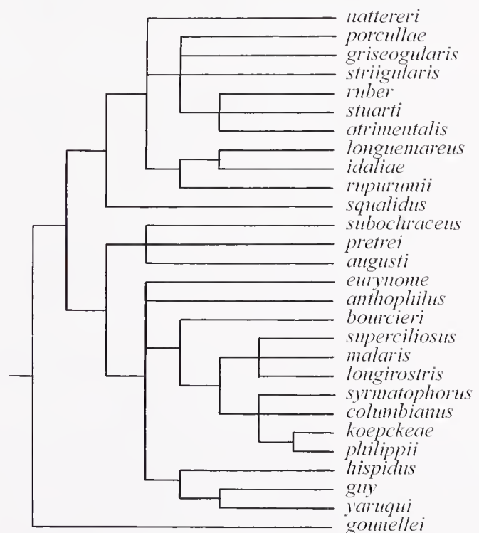
Abb. 5: Summierungsbaum von 50 der 99 gleich sparsamen Bäume; 28 Taxa, 24 Merkmale, Bewurzelung Außen-gruppe goumellei , mit und ohne Vorgabe des Kladogrammes aus Abb. 1 (Hypothesen 5 und 6 der PAUP Analysen).
