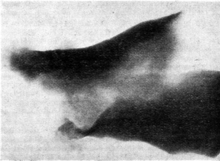
Abb. 1. Elektronenoptische Aufnahme zweier Montmorillonitteilchen aus dem „Pegmatit“ von Amberg. Teilchengröße max. 0,003 mm. Vergrößerung 45.000fach. Man beachte auch den zwischen den beiden Teilchen haftenden Flaum ( \text{SiO}_2 ).
