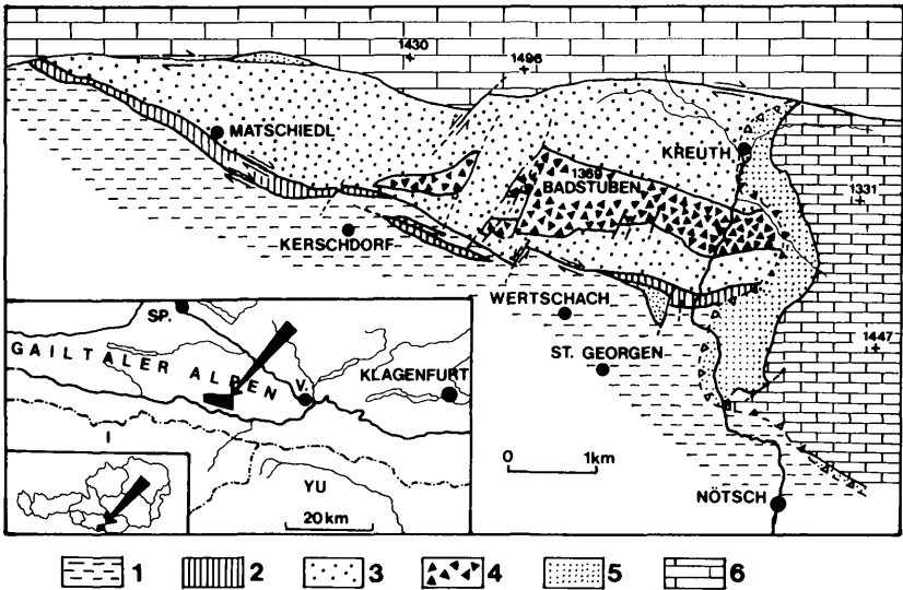
Abb. 1: Geologische Übersichtskarte des Karbon von Nötsch (nach SCHÖNLAUB 1985, stark vereinfacht). 1 Gailtalkristallin, 2 Nötscher Granitzug, 3 Karbon von Nötsch, 4 Badstubbrecie im Karbon von Nötsch, 5 Grödener Schichten und Alpiner Buntsandstein (Oberperm und unteres Skyth), 6 Karbonatensedimente der Trias.
