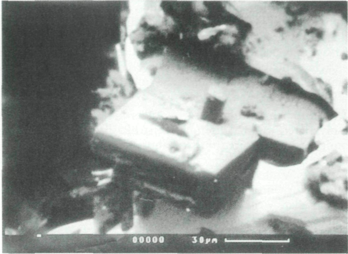
Abb. 2: Rasterelektronen- mikroskopische Aufnahme eines Chromatit-Kristall- aggregates, auf hel- ler Wulfenit-Matrix; Grube Stefanie, Bleiberg-Kreuth. Sammlung: M. PUTTNER
