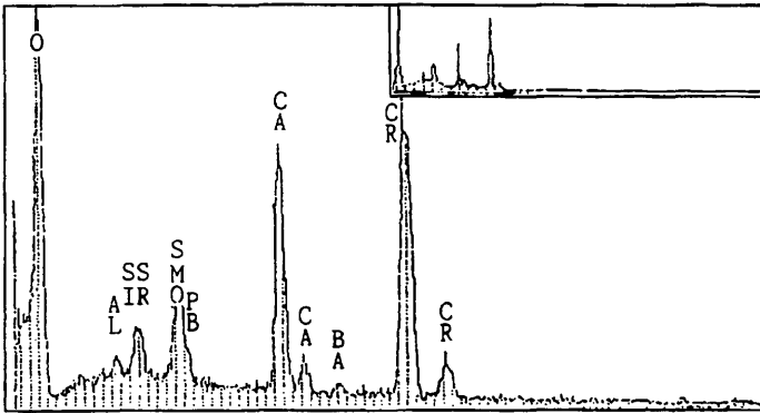
Abb. 1: EDX-Spektrum eines Chromatit- Kristalls aus Bleiberg-Kreuth.
