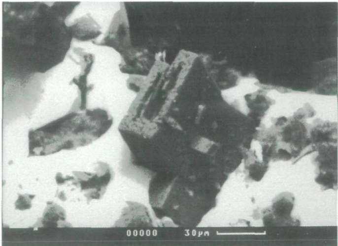
Abb. 3: Tafelige Chromatit- Kristalle aus Bleiberg-Kreuth, subparallel angeord- net; REM-Bild (Univ. d. Saar- landes).
