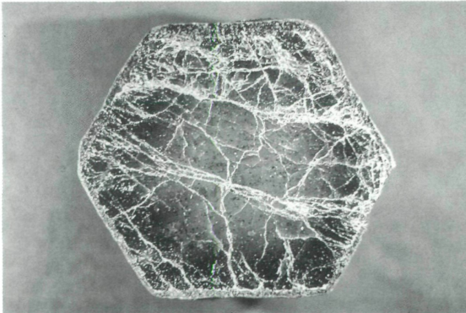
Abb. 7: Granatkristall aus dem Pusygraben bei Lölling; Neufund aus den 70-er Jahren dieses Jahrhunderts (ehemals Sammlung Johann SCHLATTE, St. Stefan bei Wolfs- berg, Kärnten). Der ca. 5,0 cm große Kristall ist geschnit- ten und poliert. Sammlung und Foto: NHM Wien (Inv.Nr. M 3310).
