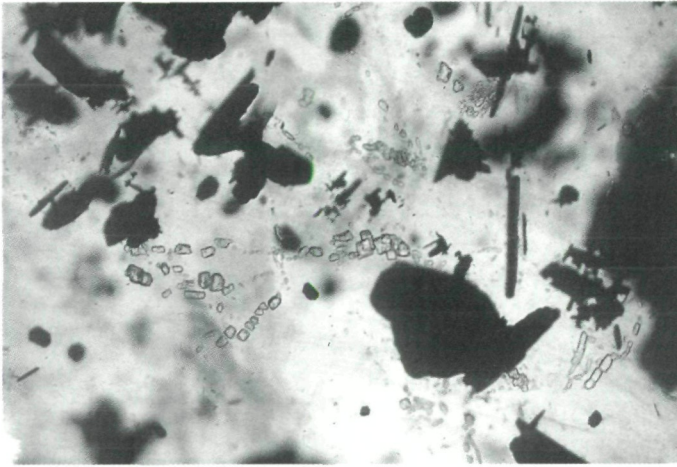
Abb. 8: Ilmenitleistchen und dichte Haufen kleiner Apatitkri- ställchen sind typisch für das Ein- schlußbild der Gra- natdase von der „Stubalpe“. Bild- breite ca. 0,3 mm.
