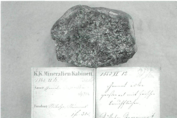
Abb. 3: Dieser etwa 10,0 x 7,0 cm große Granatkristall, mit charakteristischer Chloritrinde, wurde im vergangenen Jahrhundert noch unter der Fundortangabe „Stubalpe, Steyermark“ geführt; er stammt aber vom Unteren Grabner bei Lölling. Sammlung und Foto: NHM Wien (A.p. 732).
