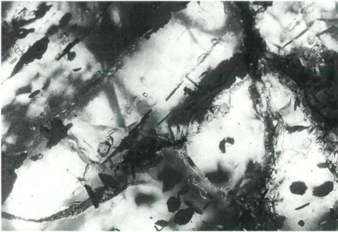
Abb. 12: Einschlüsse von Ilmenitnadeln und gelegentlich von Apatit kennzeichnen das Granatmaterial, das Herr Josef HAL- LER, Köflach, in den 70-er Jahren im Pusygraben sam- meln konnte. Foto: G. NIEDER- MAYR
