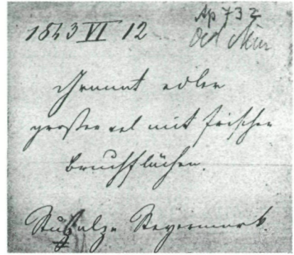
Abb. 4: Original-Etiketten zu einem Granat von der "Stubalpe, Steyermark" in der Sammlung des Naturhistorischen Museums in Wien.
