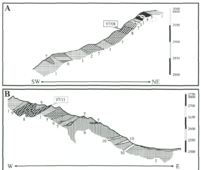
Abb. 2: Geologische Profile durch die in den beiden Untersuchungsgebieten (A: Gamsgrube, B: Großer Margrötenkopf) zutage tretenden Gesteinseinheiten (vereinfacht nach CORNELIUS & CLAR 1939).
