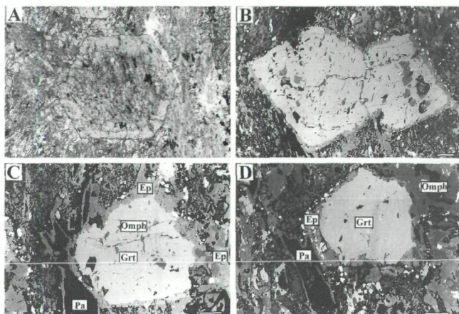
Abb. 7: A) Dünnschliffphotographie eines idiomorphen Granats (Größe: 1,5 mm) in Probe 97/08 mit Einschlussreichem Kernbereich und eher Einschlussfreiem Rand. B – C: BSE-Bilder typischer um Granat (Grt), Omphazit (Omph) und Paragonit (Pa) verlaufender Reaktionssäume aus Epidot (Ep) sowie untergeordnet aus Albit, Ca-Mg-Hornblende und Magnetit (helle Phasen in der Epidot-Corona von Bild D). Die in den Photos gezeichneten Balken entsprechen jeweils 100 Mikrometer.
