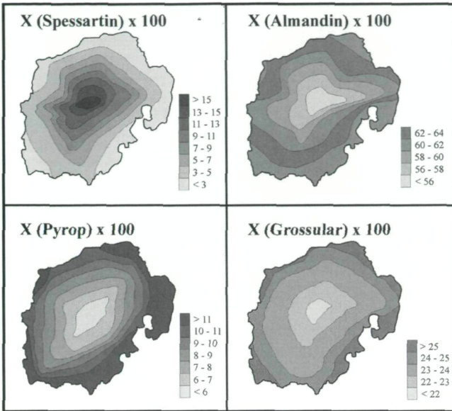
Abb. 6: Isokonzentrationskarten der vier Granatkomponenten für einen repräsentativen Kristall (Durchmesser etwa 1 mm) des eklogitischen Prasinitis im Bereich des Großen Margrözenkopfes.
