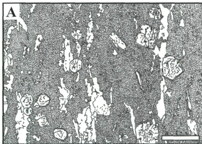
Abb. 3: Dünnschliffzeichnungen der beiden untersuchten Gesteinsproben. A) Eklogitischer Prasinit aus der Gamsgrube (97/08) mit größtenteils aus sehr feinem Symplektit bestehender Matrix, in welche die Hochdruckminerale (Granat, Paragonit, Omphazit, Na-Amphibol) eingebettet sind. B) Eklogitischer Prasinit unterhalb des Großen Margrötzenkopfes (97/11) mit symplektitischer beziehungsweise chloritischer Matrix und darin enthaltenem, reliktschen Granat, welcher deutliche Spuren eines randlichen retrograden Abbaues zeigt. Die in beiden Bildern gezeichneten Balken entsprechen jeweils 1 Millimeter.
