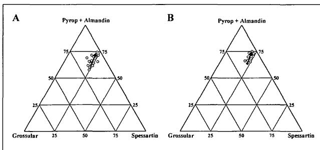
Abb. 4: Chemische Zusammen- setzung der analysierten Granate (A: Probe 97/08, B: Probe 97/11). Die in den Dreiecksdiagrammen dargestellten Punkte repräsen- tieren Kern- und Randchemismen analysierter Kristalle, während die Pfeile einen daraus resultierenden durchschnittlichen chemischen Trend vom Granatkern zum Rand zeigen.
