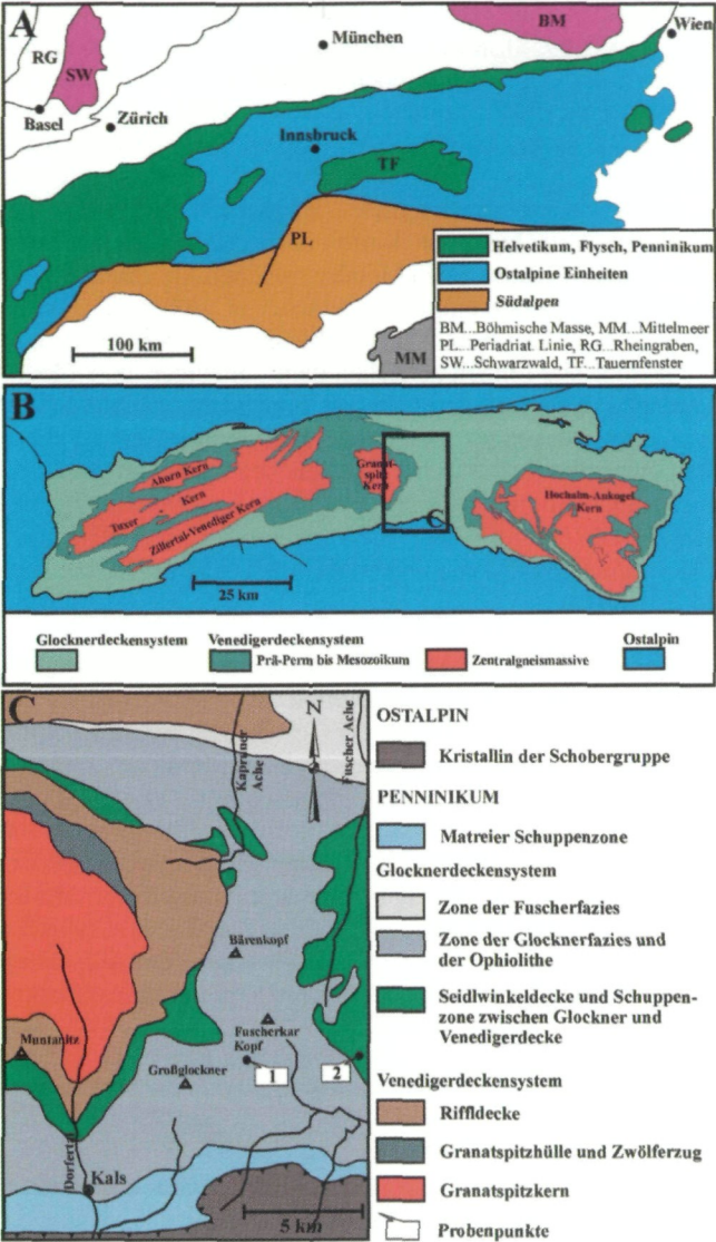
Abb. 1: A) Geologische Übersichtskarte der alpinen Großeinheiten (verändert, nach SELVERSTONE 1985) mit der Position des Penninischen Tauernfensters innerhalb des Ostalpinen Deckenkomplexes. B) Geologische Darstellung des Tauernfensters mit Gliederung in Glocknerdeckensystem (= Obere Schieferhülle) und Venedigerdeckensystem (= Zentralgneise und Untere Schieferhülle). C) Detaildarstellung des zentralen Tauernfensters laut geologischer Karte, Maßstab 1:50.000 (Blatt Grossglockner, Höck & PESTAL 1994). Änderungen der Nomenklatur und großtektonischen Zuordnung auf Basis von strukturgeologischen Ergebnissen sind bei KURZ et al. (1996) nachzulesen. Die Positionen der untersuchten Proben (1 = Probe 97/08, 2 = Probe 97/11) sind gekennzeichnet.
