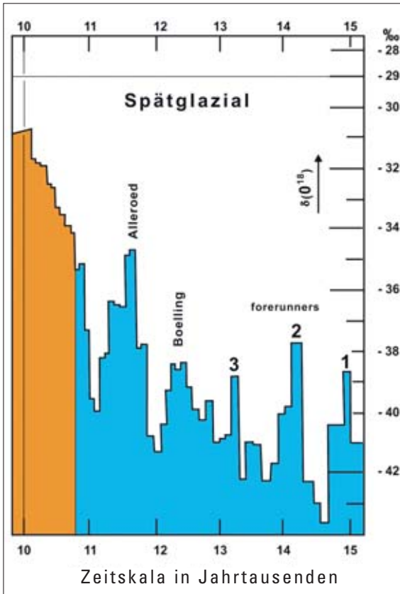
Abb. 6: Sauerstoffisotopenkurve \delta^{18}O des Eisbohrkerns Camp Century (Grönland), begrenzt auf das Spätglazial. Diagrammausschnitt aus DANSGAARD et al. 1969, Fig. 4, leicht verändert und ergänzt. (Postglazial orange, Spätglazial blau).
