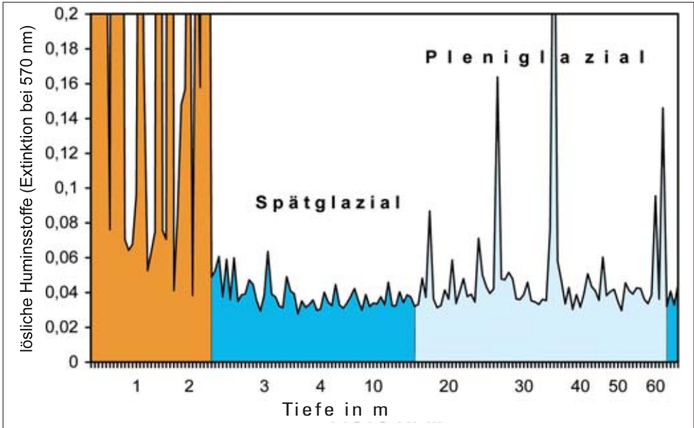
Abb. 1: Unkorrigierte Huminstoffkurve aus dem Dobramoor. Die Kurve lässt drei klimastratigraphische Bereiche erkennen, welche dem warmzeitlichen Postglazial (orange) dem kaltzeitlichen Spätglazial (dunkelblau) und dem moderat-kaltzeitlichen Lascaux-Interstadial des ausgehenden Pleniglazials (hellblau) entsprechen.
