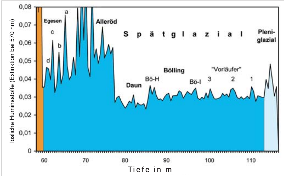
Abb. 4: Das Spätglazial im Seebachtal. Ausschnitt aus der Huminstoffkurve des Diagramms „Stappitzer See“, dargestellt in einer stark auflösenden Skalierung. Die bereits etablierten Fachausdrücke der spätglazialen Klimageschichte sind in Fettdruck gehalten. Die Bezeichnungen im Normaldruck beziehen sich auf klimatische Ereignisse, die zur Diskussion gestellt sind. Bö-I = Bölling-Initialerwärmung, Bö-H = Bölling-Höhepunkt. (Postglazial orange, Spätglazial dunkelblau, moderat-kaltzeitliches Pleni-glazial hellblau).
