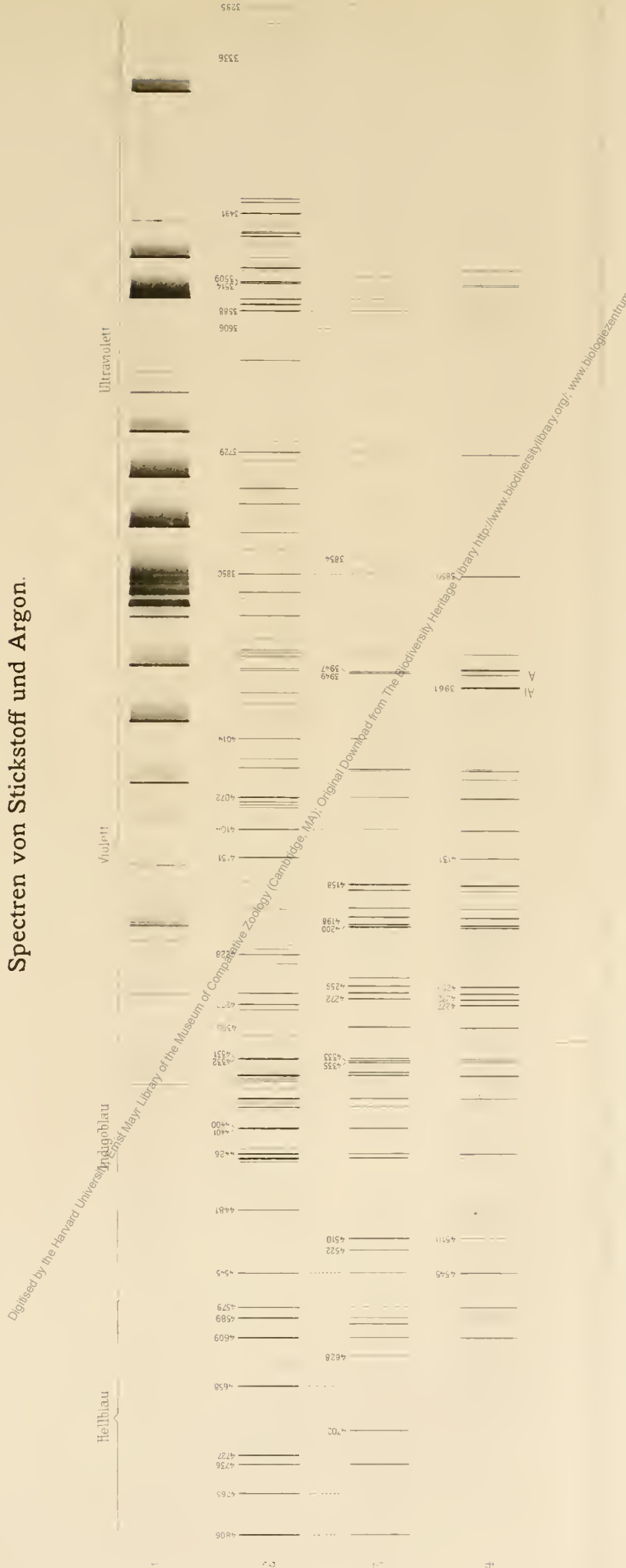
1. Bandenspectrum des Stickstoffs (3 mm Druck), ohne Flasche.
