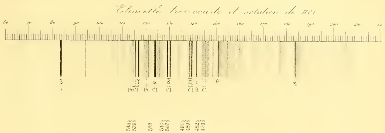
Fig. 1. Zeichnung des zwischen Platinelektroden und Salzsäure entstehenden Funkenspectrums von Lecoq.
