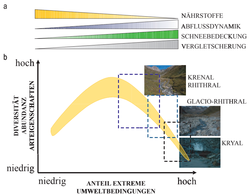
Abb. 8: Szenario der Auswirkung des Klimawandels auf Umweltfaktoren und damit auf Struktur und Funktion der Lebensgemeinschaften (hier als Diversität, Taxazahl und Variabilität von Arteigenschaften) von Gebirgsbächen (FÜREDER 2007; FÜREDER 2012, verändert).
