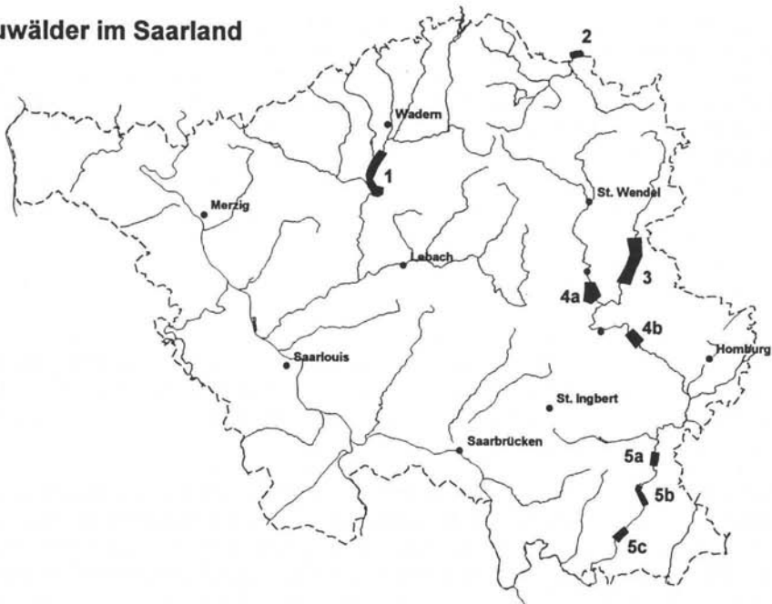
Abb. 1: Lage der Gewässerabschnitte, in denen noch Auwaldfragmente vorkommen und aufgenommen wurden
