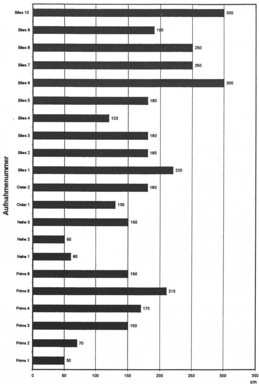
Abb.2: Niedrigwasserabstand zur Geländeoberfläche zum Zeitpunkt der Aufnahme
