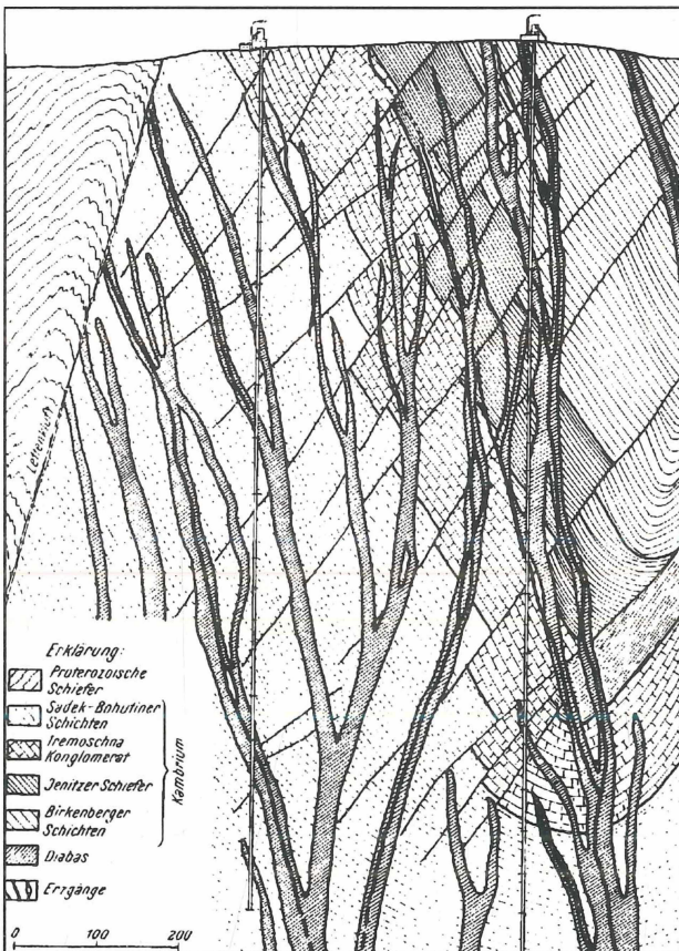
■ NW-SE-Saigerriß der Lagerstätte Pribram (nach Kettner) aus W. Petraschek – Lagerstättenlehre
