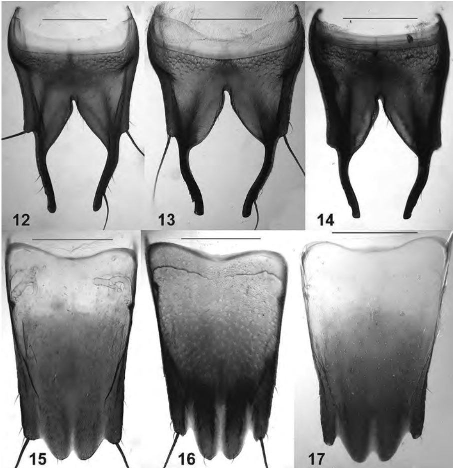
Abb. 12-17: ♂-Sternit VIII von (12) Tachinus subterraneus (LINNAEUS), Sachsen, Chemnitz; (13) Tachinus lackneri nov.sp., Holotypus; (14) Tachinus reuteri nov.sp., Holotypus; ♂-Tergit VIII von (15) Tachinus subterraneus (Linnaeus), Sachsen, Chemnitz; (16) Tachinus lackneri nov.sp., Holotypus; (17) Tachinus reuteri nov.sp., Paratypus. Alle Maßstäbe 0,5 mm.
