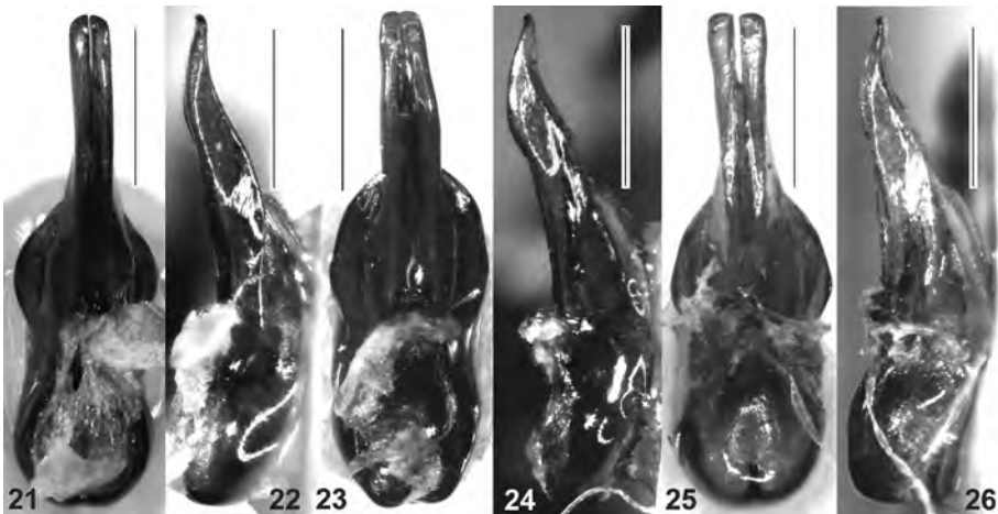
Abb. 21-26: Aedoeagus ventral (21, 23, 25) und lateral (22, 24, 26) von Tachinus subterraneus (LINNAEUS), Frankreich, Hte. Savoie (21-22); Tachinus lackneri nov.sp., Holotypus (23-24); Tachinus reuteri nov.sp., Holotypus (25-26). Alle Maßstäbe 0,5 mm.
