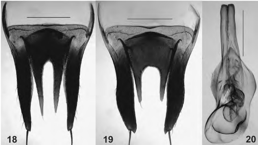
Abb. 18-20: ♀-Tergit VIII von (18) Tachinus subterraneus (Linnaeus), Brandenburg, Schorfheide; (19) Tachinus lackneri nov.sp., Paratypus; (20) Aedoeagus von Tachinus reuteri nov.sp., Paratypus ventral, im Durchlicht. Alle Maßstäbe 0,5 mm.
