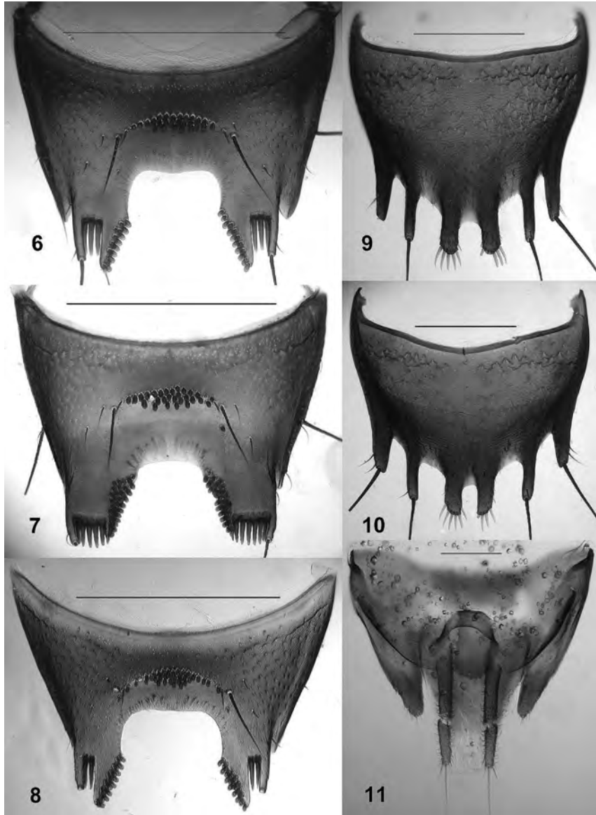
Abb. 6-11: ♂-Sternit VII von (6) Tachinus subterraneus (LINNAEUS), Sachsen, Chemnitz; (7) Tachinus lackneri nov.sp., Holotypus; (8) Tachinus reuteri nov.sp., Paratypus; ♀-Sternit VIII von (9) Tachinus subterraneus (LINNAEUS), Brandenburg, Schorfheide; (10) Tachinus lackneri nov.sp., Paratypus; (11) ♀-Segmente IX-X von Tachinus lackneri nov.sp., Paratypus. Maßstäbe 1 mm (6-8), 0,5 mm (9-10) und 0,2 mm (11).
