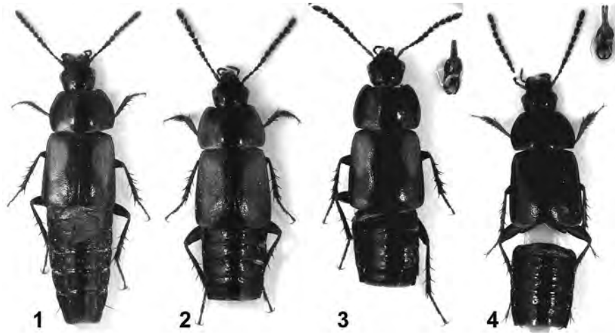
Abb. 1-4: Habitus von (1) Tachinus subterraneus (LINNAEUS), Normalfärbung, ♂ Brandenburg, Schorfheide; (2) Tachinus subterraneus (LINNAEUS), helle Färbungsvariante, ♂ Sachsen, Chemnitz; (3) Tachinus lackneri nov.sp., Holotypus-♂; (4) Tachinus reuteri nov.sp., Holotypus-♂.
